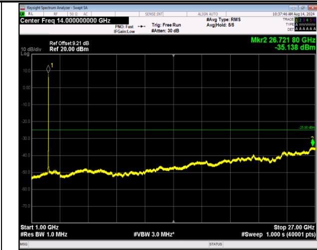
7-7-20MHz-10MHz-QPSK-QPSK-21251-21395-100RB#0-5 ORB#0-1000~27000MHz-PASS
