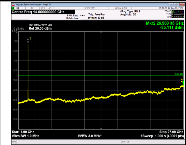
7-7-20MHz-10MHz-QPSK-QPSK-21051-21195-100RB#0-5 ORB#0-1000~27000MHz-PASS
