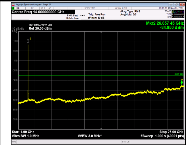
7-7-20MHz-20MHz-QPSK-QPSK-21001-21199-100RB#0-1 00RB#0-1000~27000MHz-PASS
