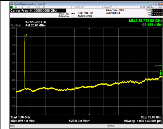
7-7-20MHz-10MHz-QPSK-QPSK-20850-20994-100RB#0-5 ORB#0-1000~27000MHz-PASS
