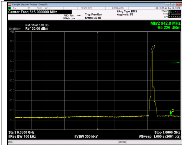
5-5-10MHz-10MHz-QPSK-QPSK-20476-20575-50RB#0-50RB#0-30~1000MHz-PASS
