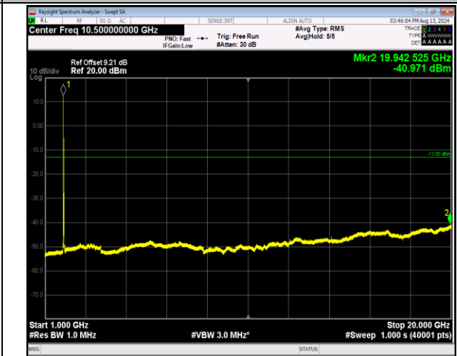
2-2-20MHz-20MHz-16QAM-16QAM-18700-18898-1RB#0-1 RB#99-1000~20000MHz-PASS
