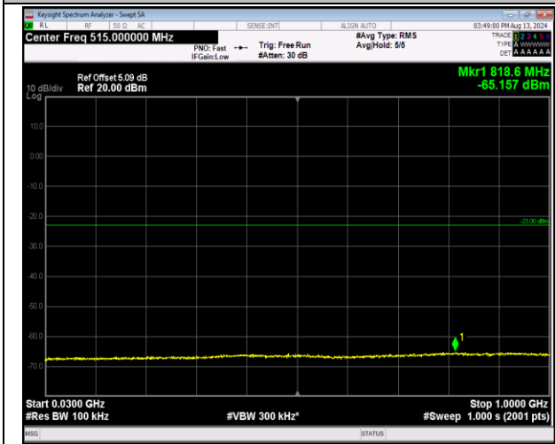
2-2-20MHz-20MHz-QPSK-QPSK-18801-18999-1RB#99-99 ORB#0-30~1000MHz-PASS
