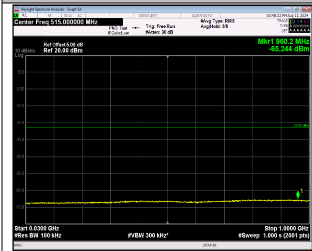
2-2-20MHz-20MHz-16QAM-16QAM-18801-18999-1RB#0 -0RB#0-30~1000MHz-PASS
