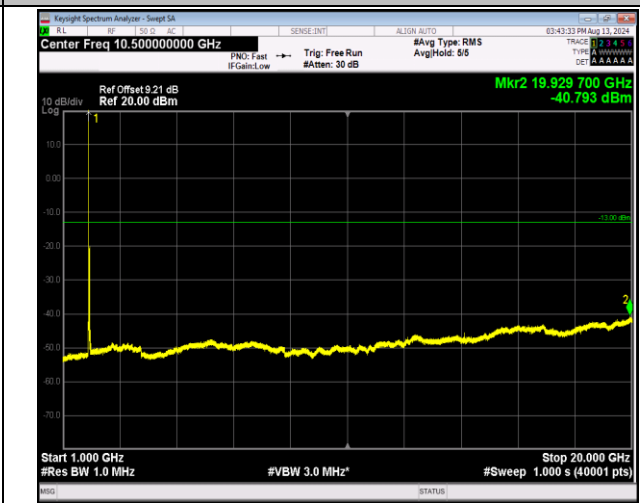
2-2-20MHz-20MHz-16QAM-16QAM-18700-18898-1RB#0-0 RB#0-1000~20000MHz-PASS
