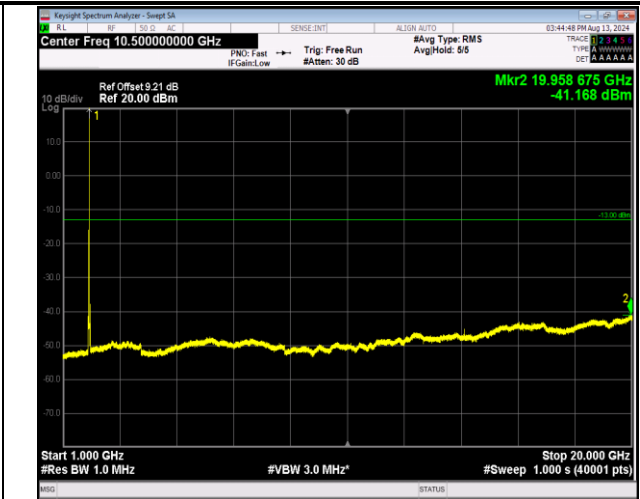
2-2-20MHz-20MHz-16QAM-16QAM-18700-18898-1RB#99- ORB#0-1000~20000MHz-PASS
