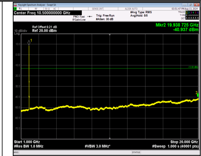
2-2-20MHz-20MHz-QPSK-QPSK-18801-18999-100RB#0-1 00RB#0-1000~20000MHz-PASS
