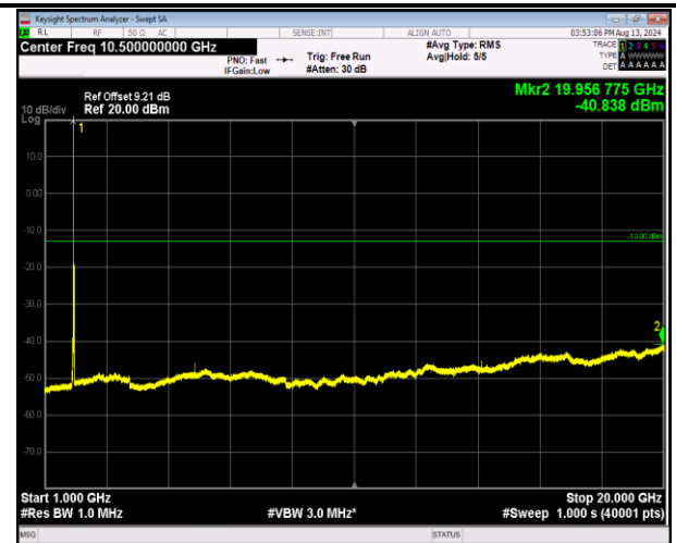
2-2-20MHz-20MHz-QPSK-QPSK-18902-19100-1RB#0-0RB #0-1000~20000MHz-PASS
