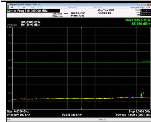
2-2-20MHz-20MHz-QPSK-QPSK-18902-19100-1RB#99-99 ORB#0-30~1000MHz-PASS
