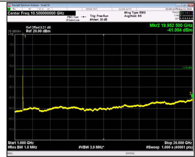
2-2-20MHz-20MHz-QPSK-QPSK-18801-18999-1RB#99-0R B#0-1000~20000MHz-PASS
