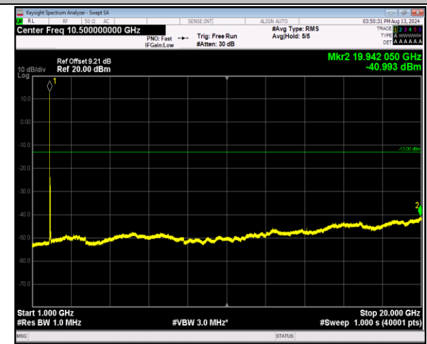
2-2-20MHz-20MHz-QPSK-QPSK-18801-18999-1RB#0-1RB #99-1000~20000MHz-PASS
