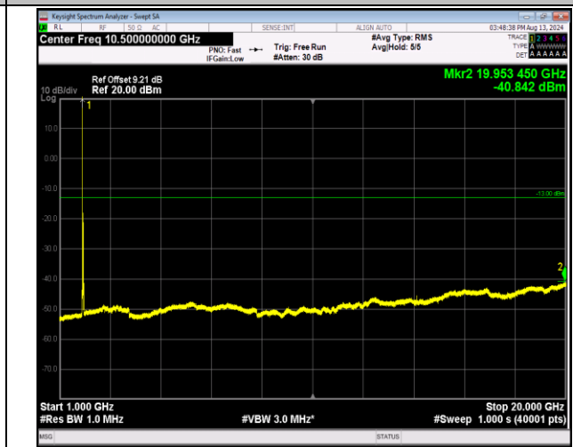
2-2-20MHz-20MHz-16QAM-16QAM-18801-18999-1RB#0-0 RB#0-1000~20000MHz-PASS
