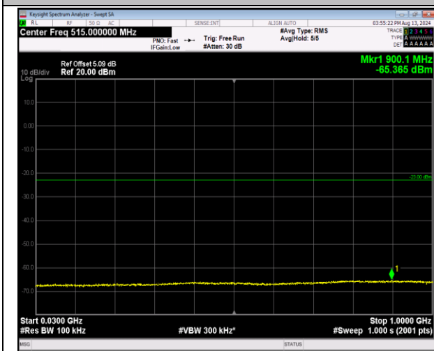
2-2-20MHz-20MHz-QPSK-QPSK-18902-19100-1RB#0-1 RB#99-30~1000MHz-PASS
