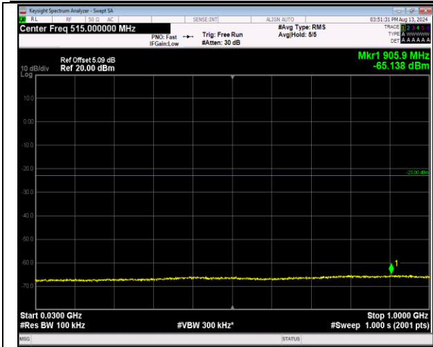
2-2-20MHz-20MHz-QPSK-QPSK-18801-18999-100RB#0 -100RB#0-30~1000MHz-PASS
