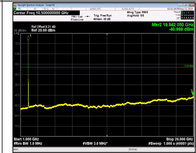
2-2-20MHz-20MHz-16QAM-16QAM-18801-18999-1RB#0-1 RB#99-1000~20000MHz-PASS
