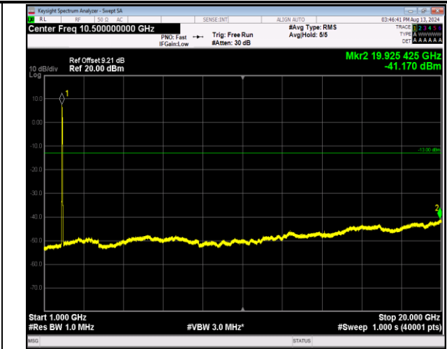
2-2-20MHz-20MHz-QPSK-QPSK-18700-18898-100RB#0-1 00RB#0-1000~20000MHz-PASS
