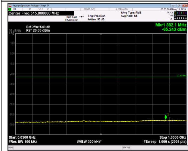
2-2-20MHz-20MHz-16QAM-16QAM-18902-19100-1RB#0 -0RB#0-30~1000MHz-PASS
