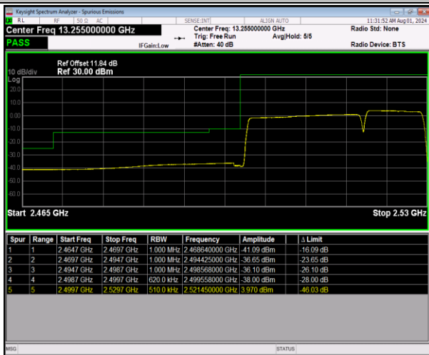
7-7-20MHz-10MHz-64QAM@64QAM-64QAM@64QAM-2
