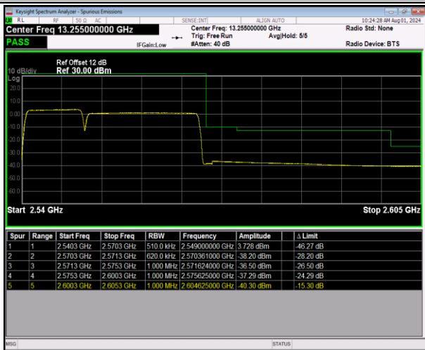
7-7-10MHz-20MHz-64QAM@64QAM-64QAM@64QAM-2
