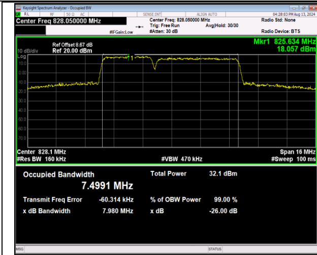
5-5-3MHz-5MHz-QPSK-QPSK-20416-20455-15RB#0-25 RB#0-PASS
