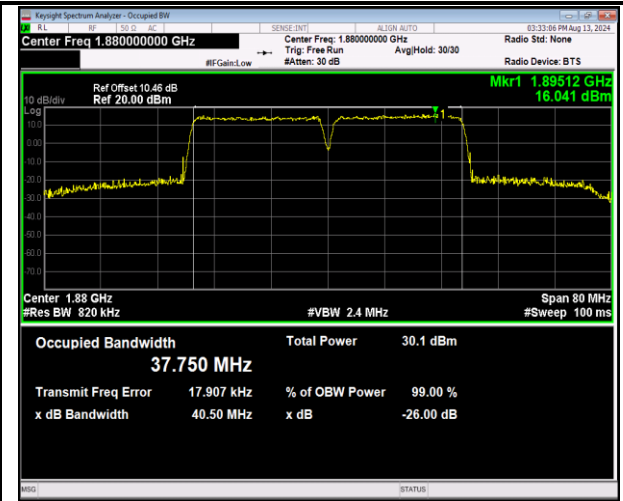
2-2-20MHz-20MHz-16QAM-16QAM-18801-18999-100RB#0-100RB#0-PASS
