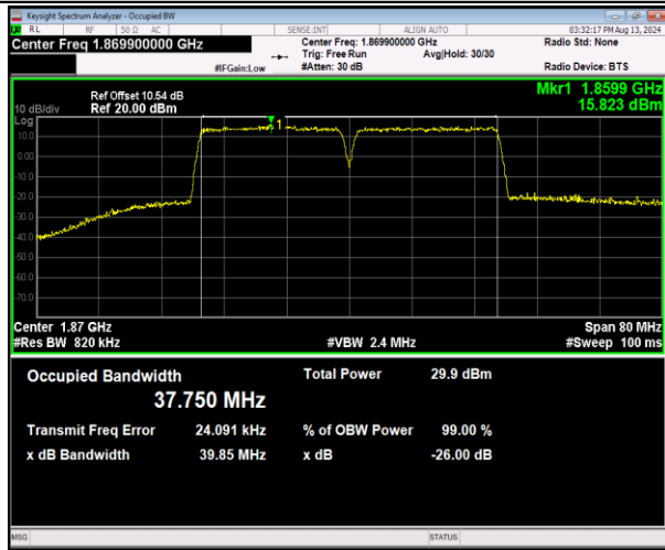
2-2-20MHz-20MHz-16QAM-16QAM-18700-18898-100RB#0-100RB#0-PASS
