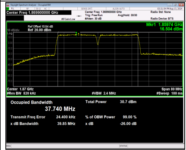
2-2-20MHz-20MHz-QPSK-QPSK-18700-18898-100RB#0-100RB#0-PASS
