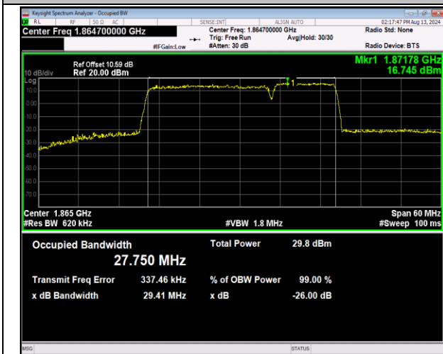
2-2-20MHz-10MHz-16QAM-16QAM-18700-18844-100RB #0-50RB#0-PASS
