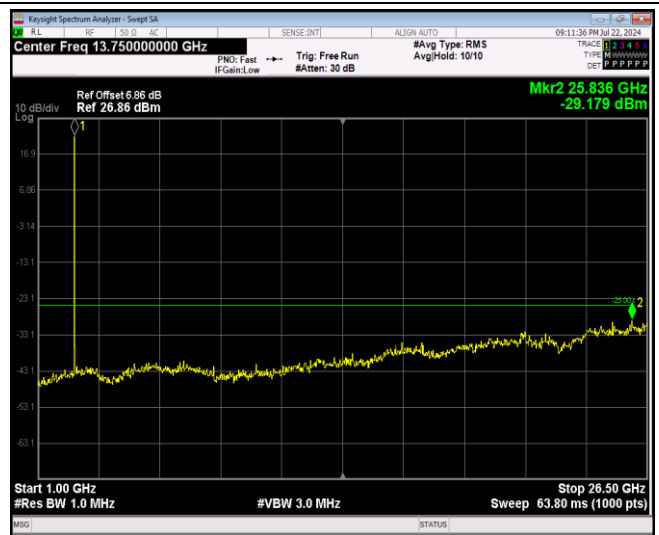
Band41-5MHz-QPSK-40640-1RB#0-Range2:1000~265 00MHz
