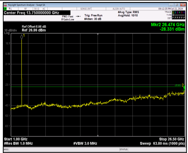
Band41-5MHz-QPSK-41215-1RB#0-Range2:1000~265 00MHz
