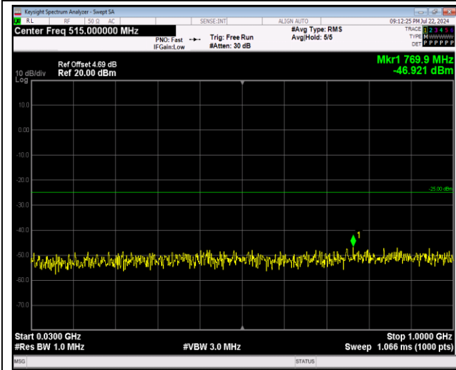
Band41-5MHz-QPSK-41215-1RB#0-Range1:30~100 OMHz
