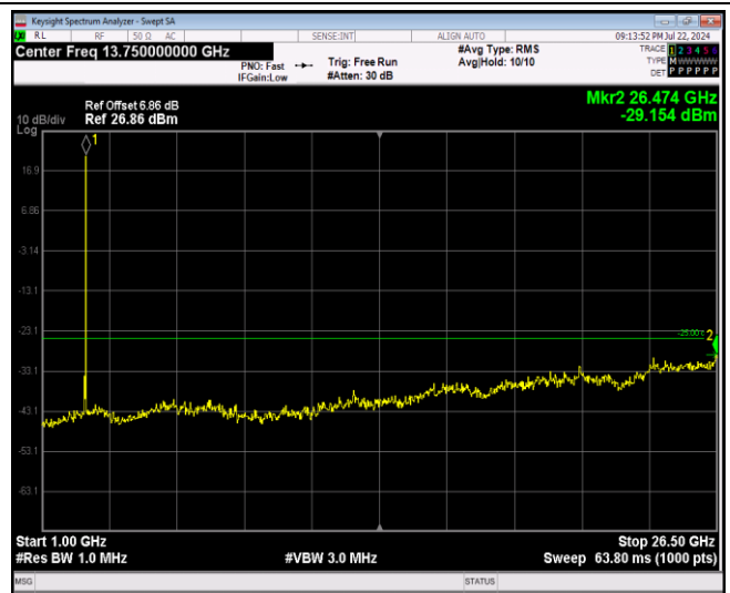
Band41-5MHz-64QAM-40065-1RB#0-Range2:1000~26500MHz
