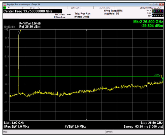
Band7-20MHz-QPSK-21100-1RB#0-Range2:1000~265 00MHz
