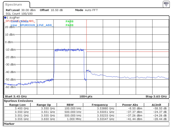
40MHz_30kHz_3530MHz_DFT-s-OFDM QPSK_RB100@0 -37.26 dBm
