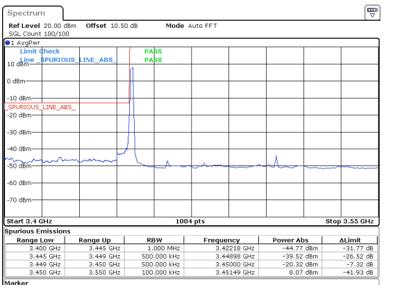
60MHz_30kHz_3480MHz_DFT-s-OFDM QPSK_RB1@0 -20.32 dBm
