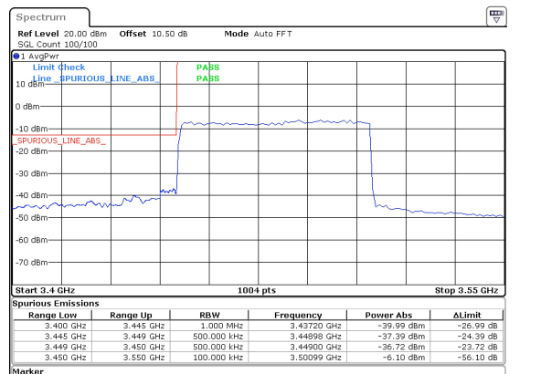
60MHz_30kHz_3480MHz_DFT-s-OFDM QPSK_RB162@0 -36.72 dBm
