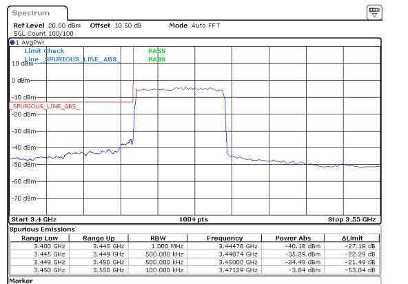
40MHz_30kHz_3470MHz_DFT-s-OFDM QPSK_RB100@0 -34.49 dBm
