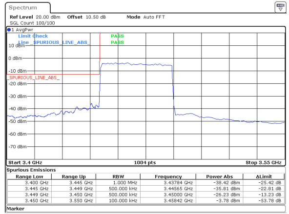
40MHz_15kHz_3470MHz_DFT-s-OFDM QPSK_RB216@0 -26.23 dBm
