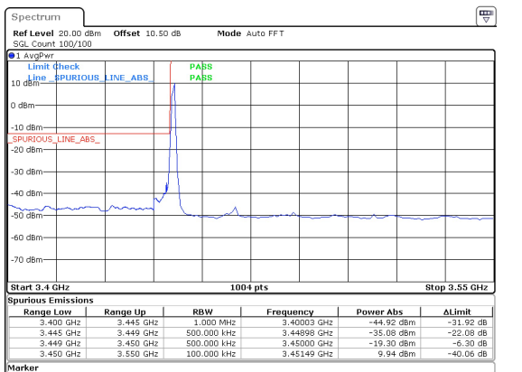
40MHz_30kHz_3470MHz_DFT-s-OFDM QPSK_RB1@0 -19.30 dBm
