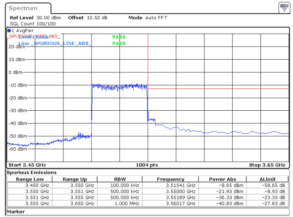
40MHz_15kHz_3530MHz_DFT-s-OFDM QPSK_RB216@0 -21.93 dBm
