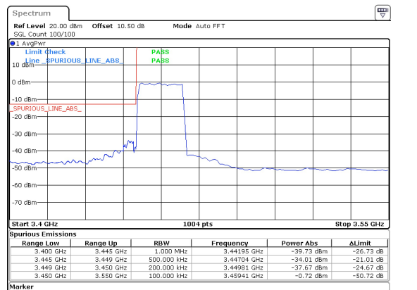
20MHz_30kHz_3460MHz_DFT-s-OFDM QPSK_RB50@0 -34.01 dBm
