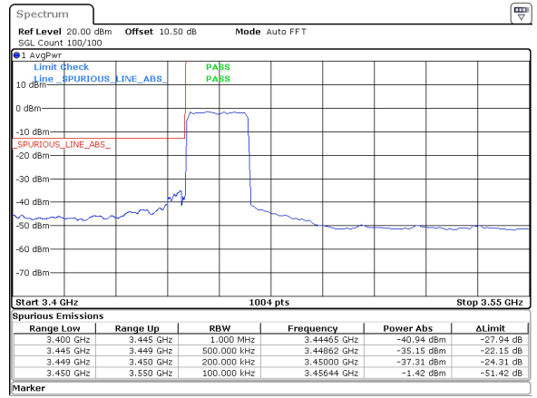
20MHz_15kHz_3460MHz_DFT-s-OFDM QPSK_RB100@0 -35.15 dBm
