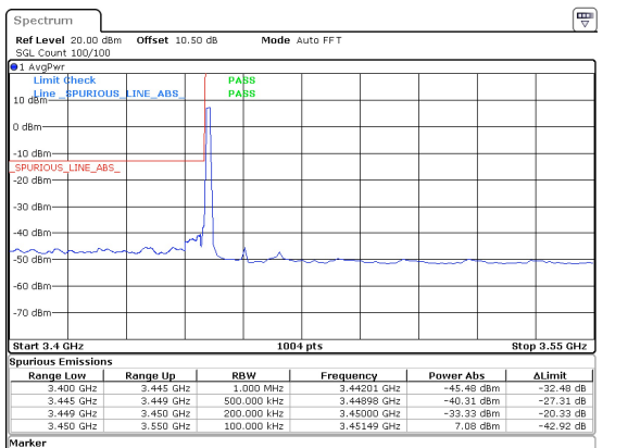
20MHz_30kHz_3460MHz_DFT-s-OFDM QPSK_RB1@0 -33.33 dBm
