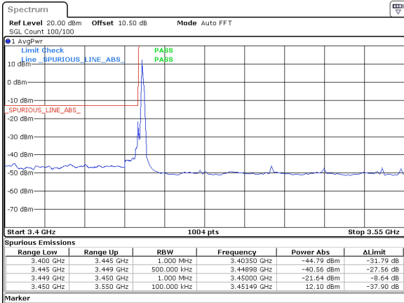
100MHz_30kHz_3500MHz_DFT-s-OFDM QPSK_RB1@0 -21.64 dBm
