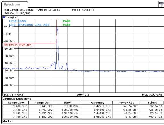
10MHz_30kHz_3455MHz_DFT-s-OFDM QPSK_RB1@0 -38.06 dBm
