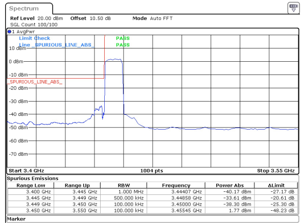
10MHz_15kHz_3455MHz_DFT-s-OFDM QPSK_RB50@0 -33.61 dBm
