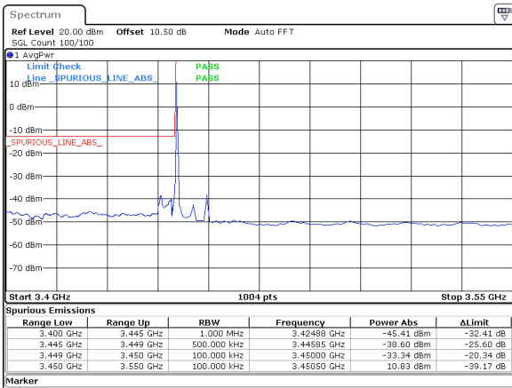
10MHz_15kHz_3455MHz_DFT-s-OFDM QPSK_RB1@0 -33.34 dBm
