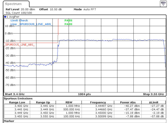
100MHz_30kHz_3500MHz_DFT-s-OFDM QPSK_RB270@0 -15.19 dBm
