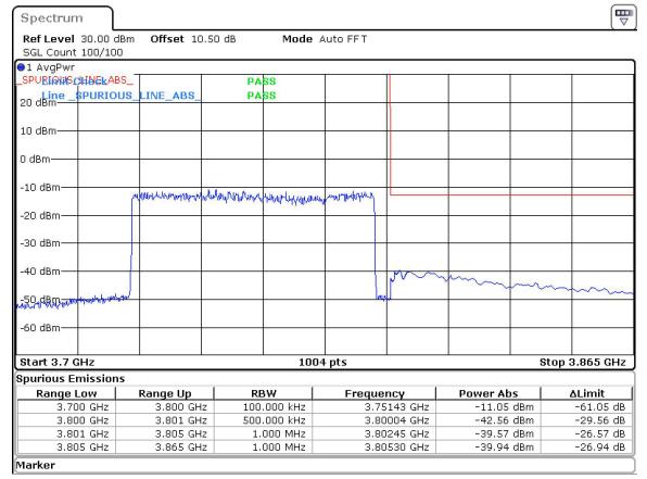
70MHz_30kHz_3765MHz_DFT-s-OFDM QPSK_RB180@0&-39.57 dBm
