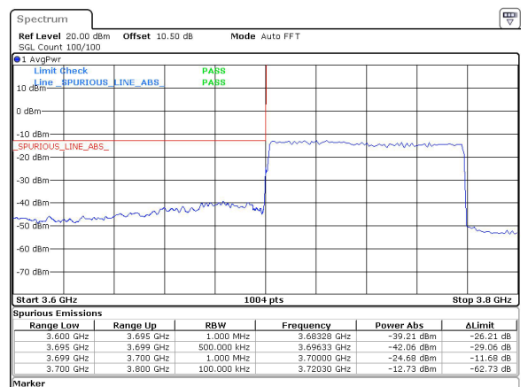
80MHz_30kHz_3740MHz_DFT-s-OFDM QPSK_RB216@0&-24.68 dBm
