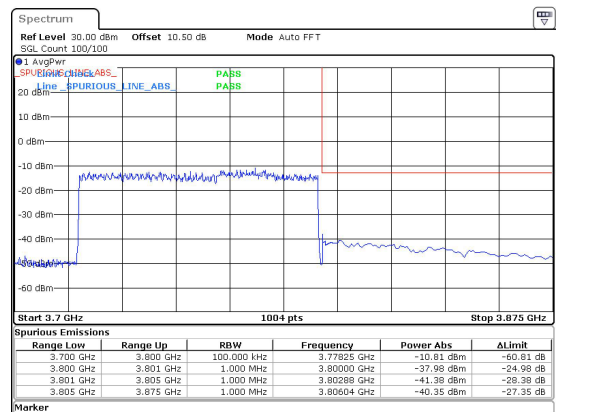
80MHz_30kHz_3760MHz_DFT-s-OFDM QPSK_RB216@0&-37.98 dBm
