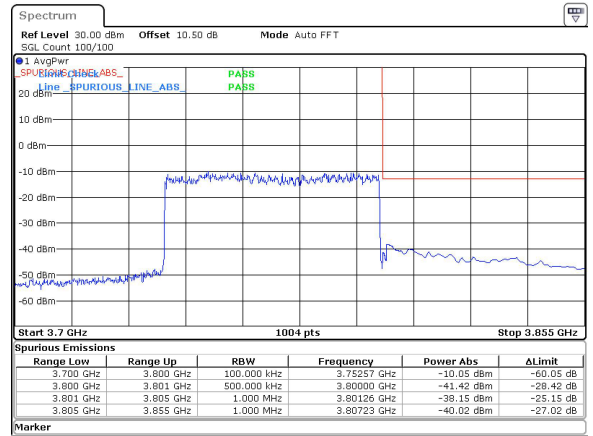
60MHz_30kHz_3770MHz_DFT-s-OFDM QPSK_RB162@0&-38.15 dBm
