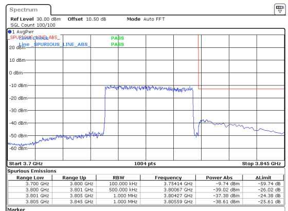
50MHz_30kHz_3775MHz_DFT-s-OFDM QPSK_RB128@0&-37.38 dBm
