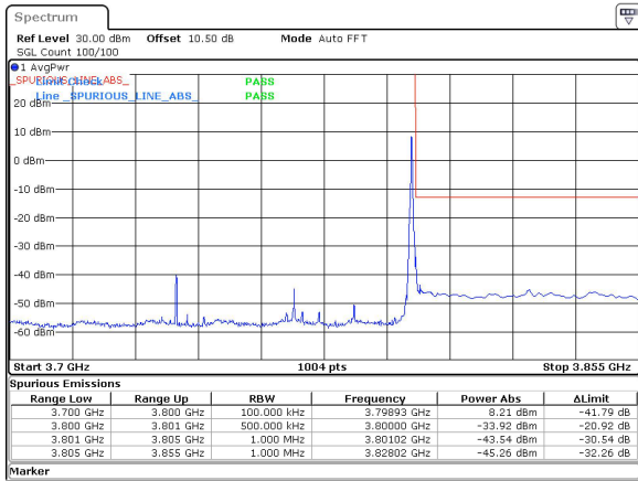
60MHz_30kHz_3770MHz_DFT-s-OFDM QPSK_RB1@161&-33.92 dBm
