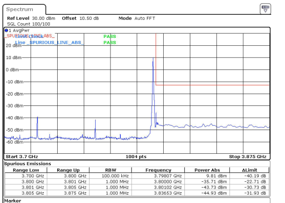
80MHz_30kHz_3760MHz_DFT-s-OFDM QPSK_RB1@216&-35.71 dBm
