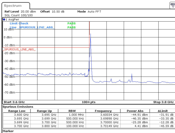
50MHz_30kHz_3725MHz_DFT-s-OFDM QPSK_RB1@0&-25.28 dBm
