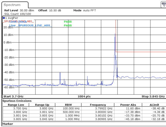
50MHz_15kHz_3775MHz_DFT-s-OFDM QPSK_RB1@269&-17.38 dBm
