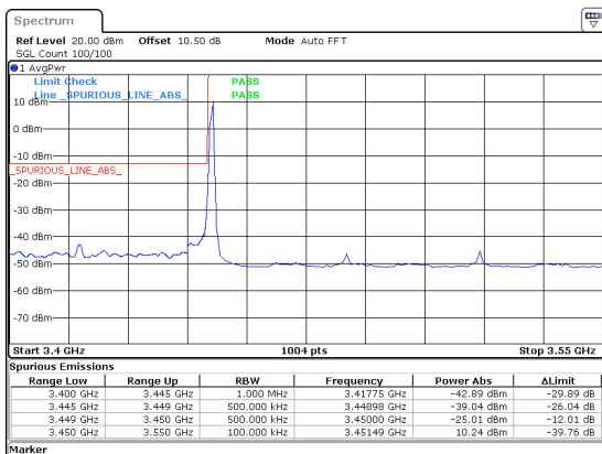
70MHz_30kHz_3485MHz_DFT-s-OFDM QPSK_RB1@0&-25.01 dBm
