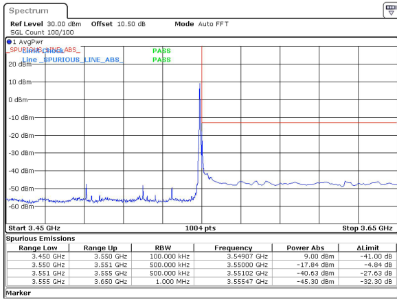
60MHz_30kHz_3520MHz_DFT-s-OFDM QPSK_RB1@161&-17.84 dBm
