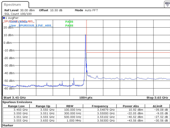
30MHz_30kHz_3535MHz_DFT-s-OFDM QPSK_RB1@77&-22.05 dBm
