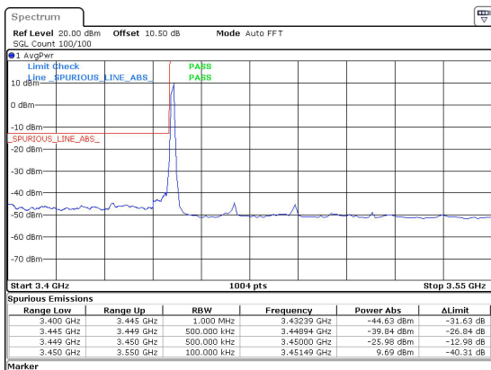
40MHz_30kHz_3470MHz_DFT-s-OFDM QPSK_RB1@0&-25.98 dBm
