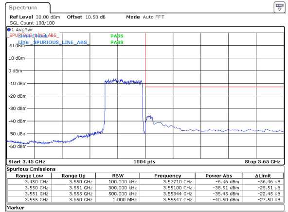
30MHz_30kHz_3535MHz_DFT-s-OFDM QPSK_RB75@0&-35.45 dBm
