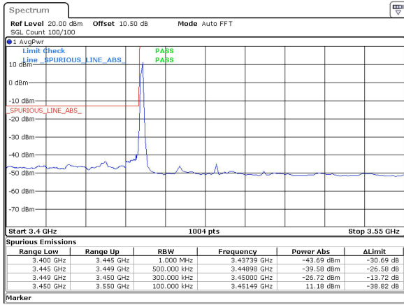
30MHz_30kHz_3465MHz_DFT-s-OFDM QPSK_RB1@0&-26.72 dBm
