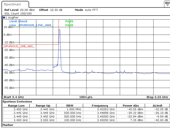
60MHz_30kHz_3480MHz_DFT-s-OFDM QPSK_RB1@0&-22.84 dBm
