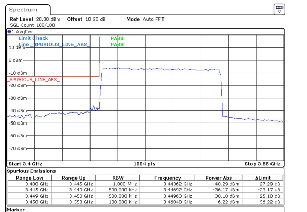
70MHz_30kHz_3485MHz_DFT-s-OFDM QPSK_RB180@0&-36.17 dBm
