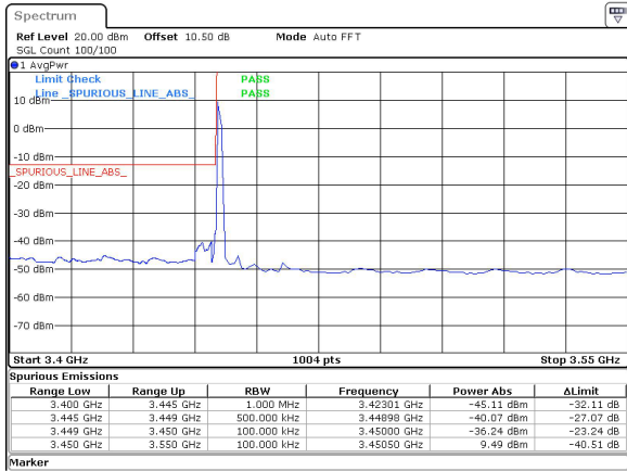
10MHz_30kHz_3455MHz_DFT-s-OFDM QPSK_RB1@0&-36.24 dBm
