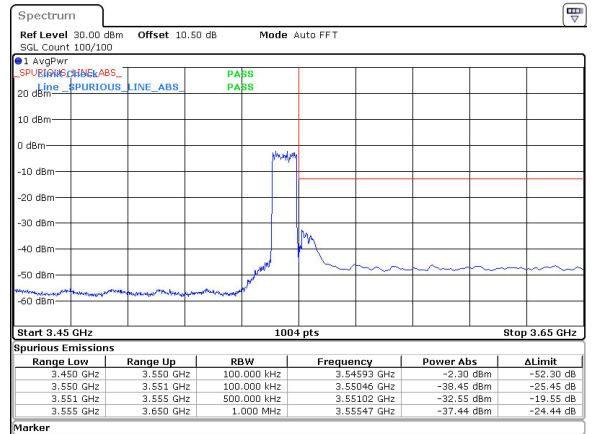
10MHz_30kHz_3545MHz_DFT-s-OFDM QPSK_RB24@0&-32.55 dBm
