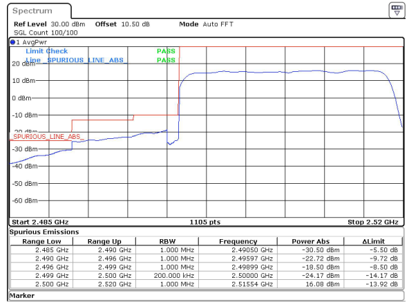
20MHz_15kHz_2510MHz_DFT-s-OFDM QPSK_RB100@0&-30.50 dBm
