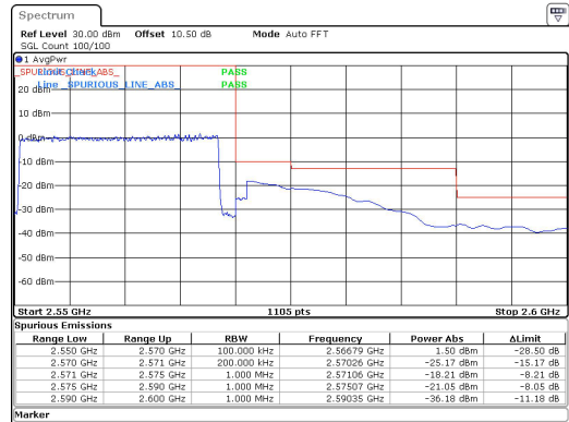
20MHz_15kHz_2560MHz_DFT-s-OFDM QPSK_RB100@0&-21.05 dBm
