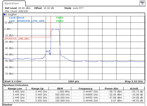
10MHz_30kHz_3455MHz_DFT-s-OFDM QPSK_RB24@0&-32.86 dBm
