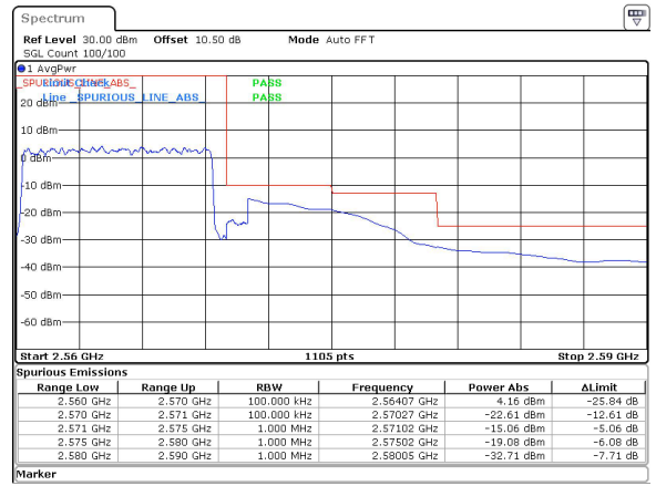
10MHz_15kHz_2565MHz_DFT-s-OFDM QPSK_RB50@0&-15.06 dBm
