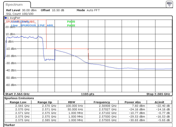
5MHz_15kHz_2567.5MHz_DFT-s-OFDM QPSK_RB25@0&-10.77 dBm
