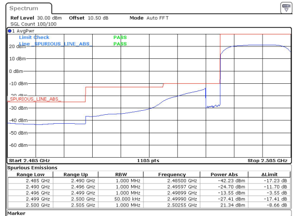
5MHz_15kHz_2502.5MHz_DFT-s-OFDM QPSK_RB25@0&-13.55 dBm
