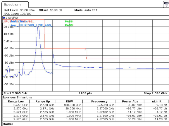
5MHz_15kHz_2567.5MHz_DFT-s-OFDM QPSK_RB1@24&-14.17 dBm
