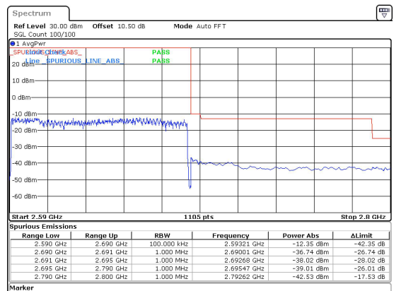
100MHz_30kHz_2640MHz_DFT-s-OFDM QPSK_RB270@0&-42.53 dBm
