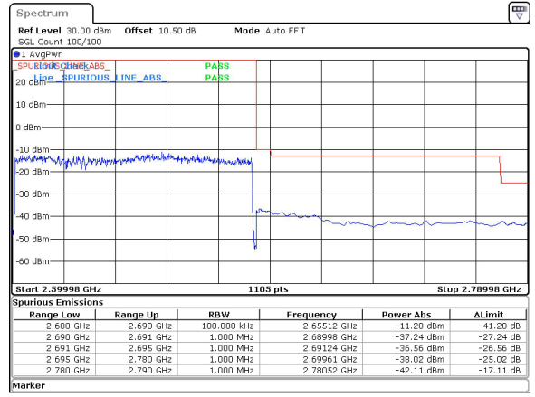
90MHz_30kHz_2644.98MHz_DFT-s-OFDM QPSK_RB243@0&-42.11 dBm
