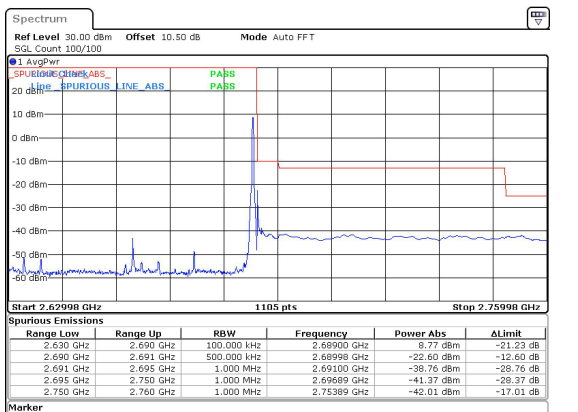
60MHz_30kHz_2659.98MHz_DFT-s-OFDM QPSK_RB1@161&-22.60 dBm
