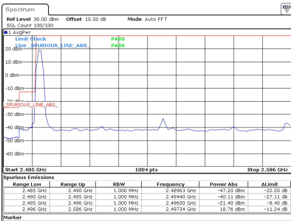
90MHz_30kHz_2541MHz_DFT-s-OFDM QPSK_RB1@0&-21.40 dBm
