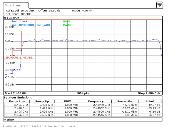
90MHz_30kHz_2541MHz_DFT-s-OFDM QPSK_RB243@0&-18.10 dBm
