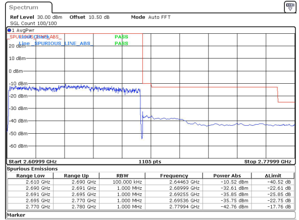
80MHz_30kHz_2649.99MHz_DFT-s-OFDM QPSK_RB216@0&-42.76 dBm
