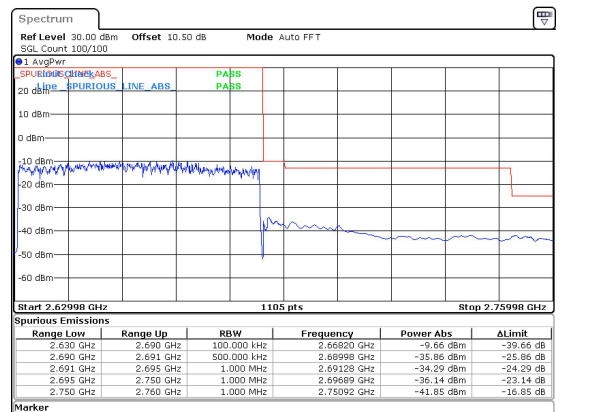
60MHz_30kHz_2659.98MHz_DFT-s-OFDM QPSK_RB162@0&-41.85 dBm
