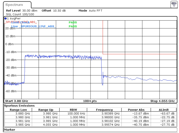
80MHz_30kHz_3940MHz_DFT-s-OFDM QPSK_RB216@0 -35.75 dBm
