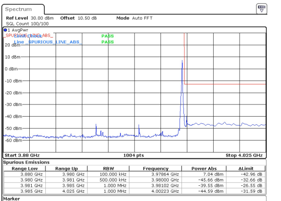
50MHz_30kHz_3955MHz_DFT-s-OFDM QPSK_RB1@132 -39.55 dBm
