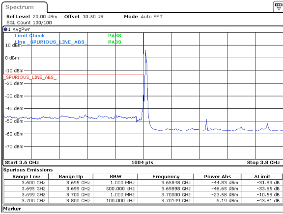
90MHz_30kHz_3745MHz_DFT-s-OFDM QPSK_RB1@0 -23.58 dBm
