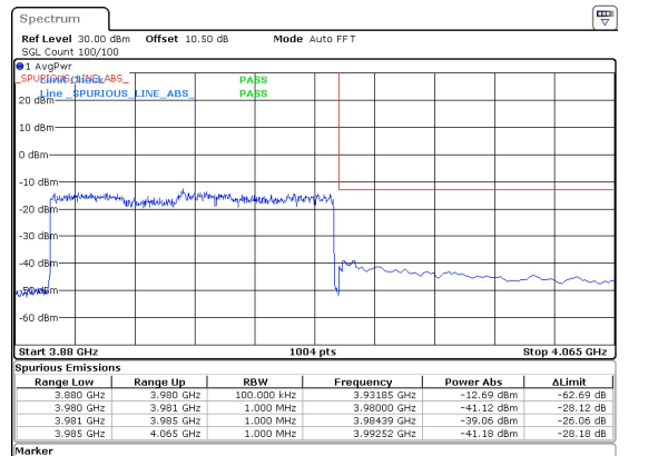
90MHz_30kHz_3935MHz_DFT-s-OFDM QPSK_RB243@0 -39.06 dBm
