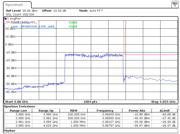
50MHz_15kHz_3955MHz_DFT-s-OFDM QPSK_RB270@0 -39.58 dBm
