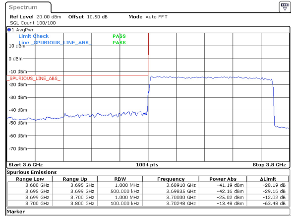
90MHz_30kHz_3745MHz_DFT-s-OFDM QPSK_RB243@0 -25.02 dBm
