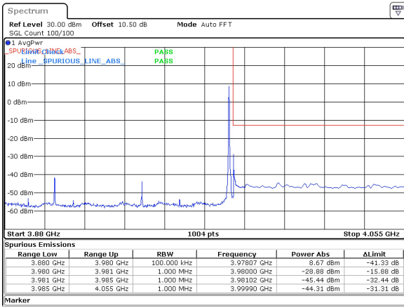
80MHz_30kHz_3940MHz_DFT-s-OFDM QPSK_RB1@216 -28.88 dBm
