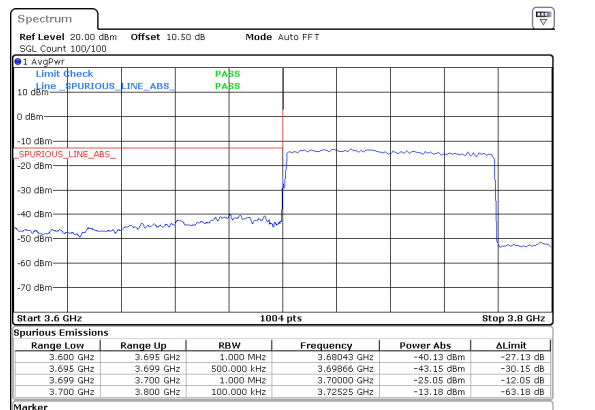
80MHz_30kHz_3740MHz_DFT-s-OFDM QPSK_RB216@0 -25.05 dBm
