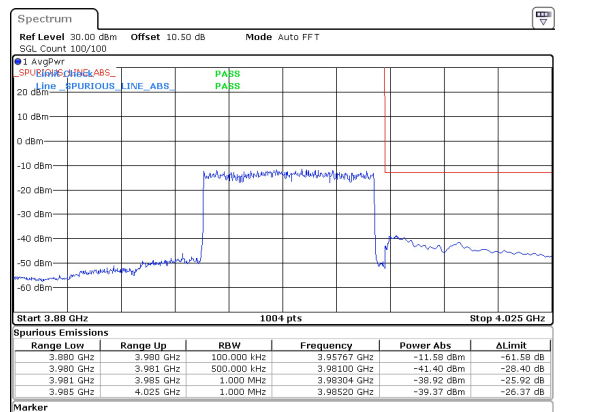
50MHz_30kHz_3955MHz_DFT-s-OFDM QPSK_RB128@0 -38.92 dBm
