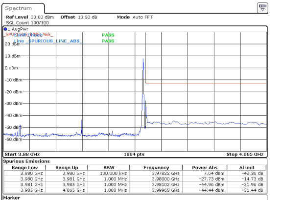
90MHz_30kHz_3935MHz_DFT-s-OFDM QPSK_RB1@244 -27.73 dBm
