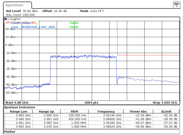
60MHz_30kHz_3950MHz_DFT-s-OFDM QPSK_RB162@0 -39.96 dBm
