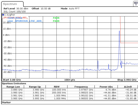
20MHz_30kHz_3970MHz_DFT-s-OFDM QPSK_RB1@50 -41.51 dBm
