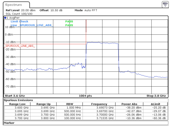
40MHz_15kHz_3720MHz_DFT-s-OFDM QPSK_RB216@0 -26.06 dBm
