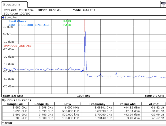
40MHz_30kHz_3720MHz_DFT-s-OFDM QPSK_RB1@0 -42.99 dBm
