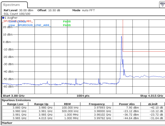
40MHz_30kHz_3960MHz_DFT-s-OFDM QPSK_RB1@105 -23.12 dBm
