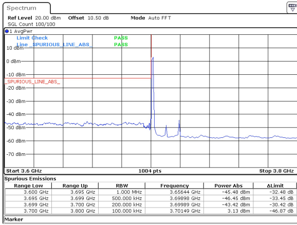
20MHz_30kHz_3710MHz_DFT-s-OFDM QPSK_RB1@0 -43.42 dBm
