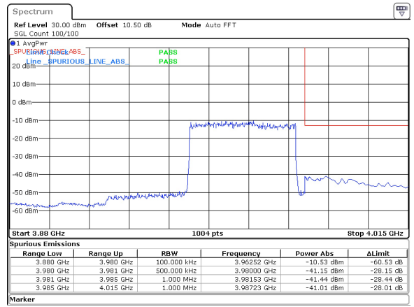
40MHz_30kHz_3960MHz_DFT-s-OFDM QPSK_RB100@0 -41.01 dBm
