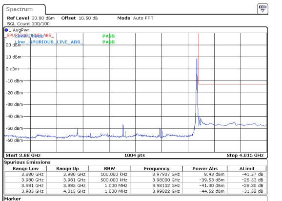
40MHz_15kHz_3960MHz_DFT-s-OFDM QPSK_RB1@215 -39.53 dBm
