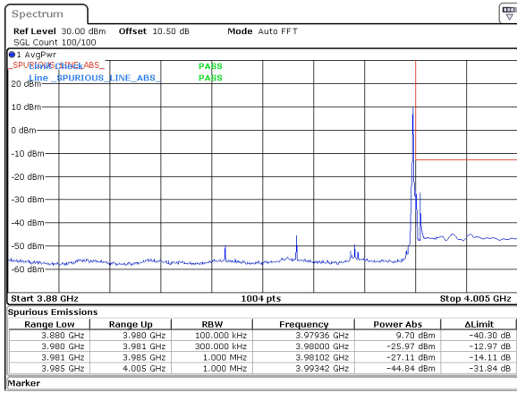
30MHz_15kHz_3965MHz_DFT-s-OFDM QPSK_RB1@159 -25.97 dBm
