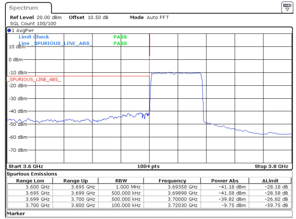
40MHz_30kHz_3720MHz_DFT-s-OFDM QPSK_RB100@0 -39.82 dBm
