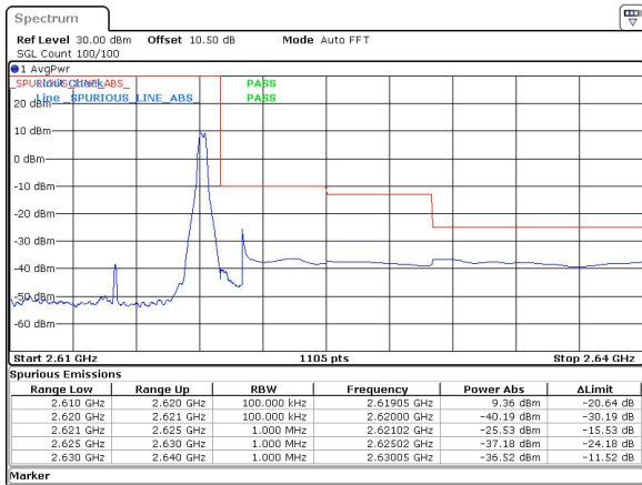
10MHz_30kHz_2615MHz_DFT-s-OFDM QPSK_RB1@23&-36.52 dBm
