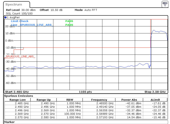
10MHz_30kHz_2575MHz_DFT-s-OFDM QPSK_RB24@0&14.54 dBm
