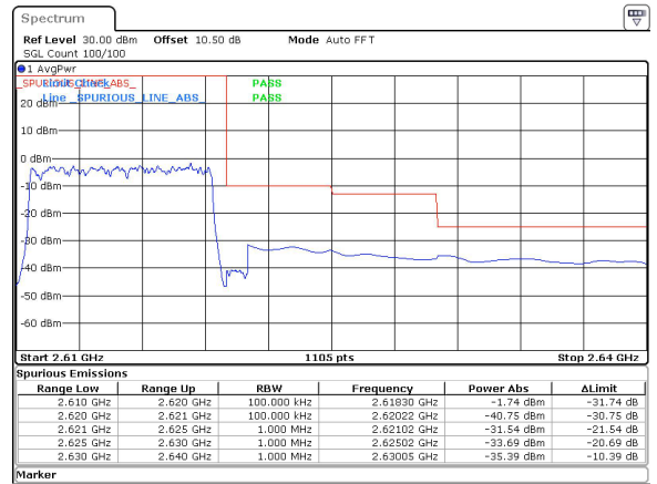
10MHz_30kHz_2615MHz_DFT-s-OFDM QPSK_RB24@0&-35.39 dBm
