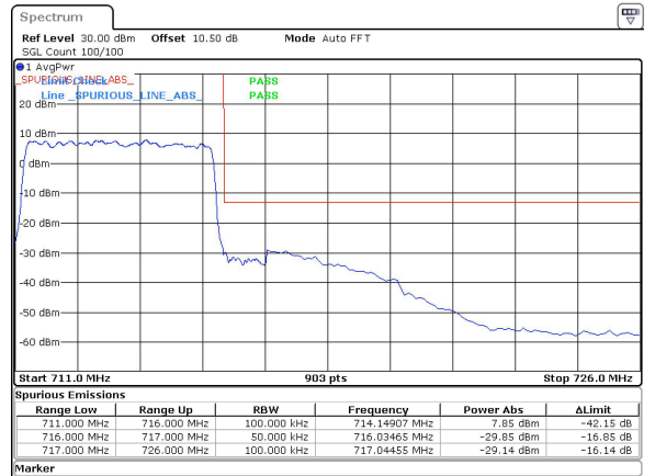
5MHz_15kHz_713.5MHz_DFT-s-OFDM QPSK_RB25@0&-29.14 dBm
