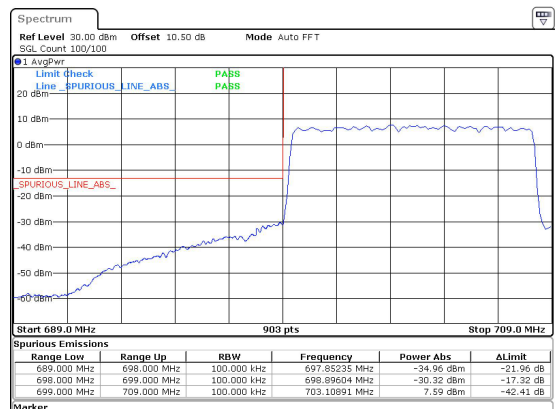
10MHz_15kHz_704MHz_DFT-s-OFDM QPSK_RB50@0&-30.32 dBm
