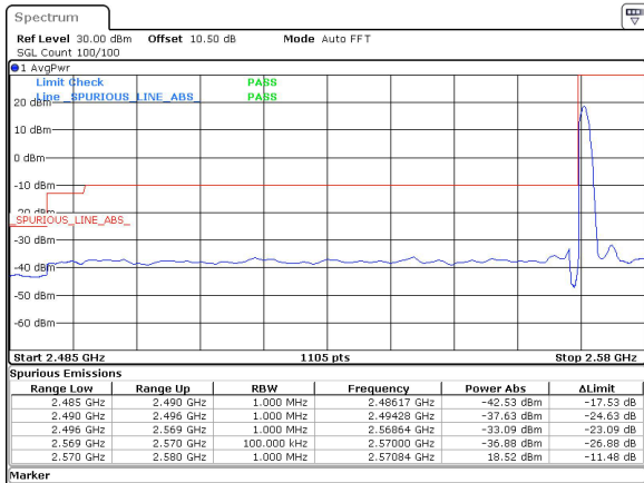
10MHz_30kHz_2575MHz_DFT-s-OFDM QPSK_RB1@0&18.52 dBm
