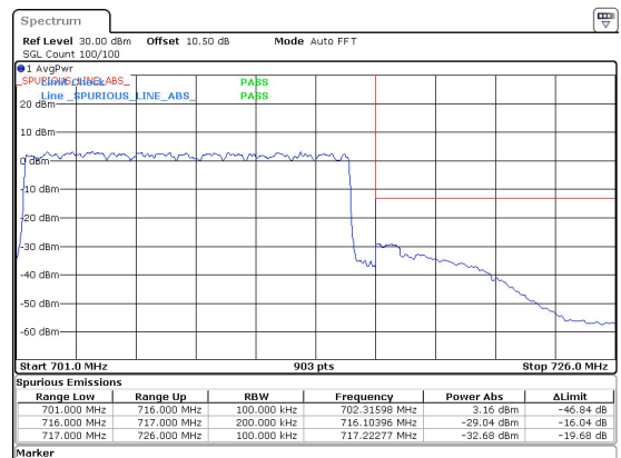
15MHz_15kHz_708.5MHz_DFT-s-OFDM QPSK_RB75@0&-29.04 dBm
