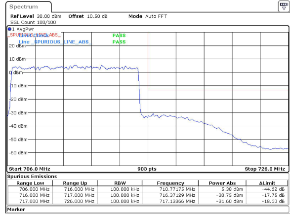
10MHz_15kHz_711MHz_DFT-s-OFDM QPSK_RB50@0&-30.75 dBm
