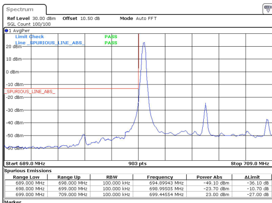
10MHz_15kHz_704MHz_DFT-s-OFDM QPSK_RB1@0&-23.70 dBm
