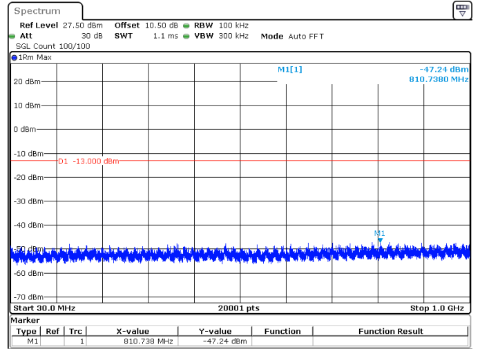
20MHz_15kHz_1770MHz_DFT-s-OFDM QPSK_RB1@105 -47.24 dBm
