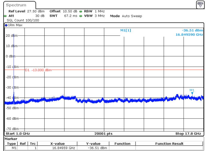
20MHz_15kHz_1770MHz_DFT-s-OFDM QPSK_RB1@0 -36.51 dBm
