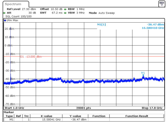
20MHz_15kHz_1720MHz_DFT-s-OFDM QPSK_RB1@0 -36.47 dBm
