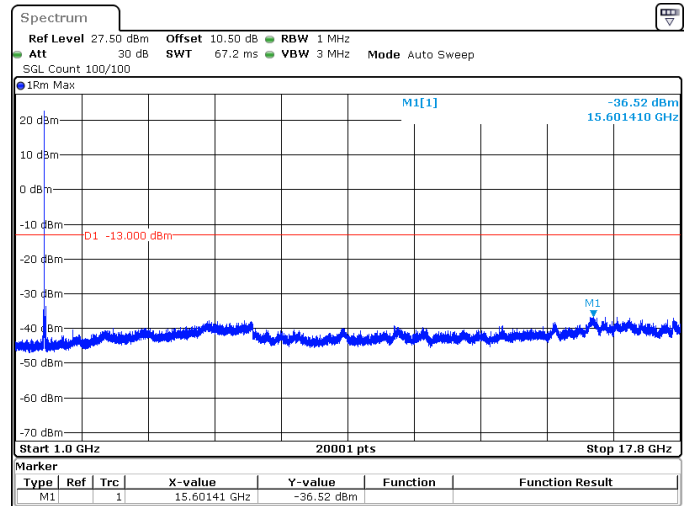
20MHz_15kHz_1720MHz_DFT-s-OFDM QPSK_RB1@105 -36.52 dBm
