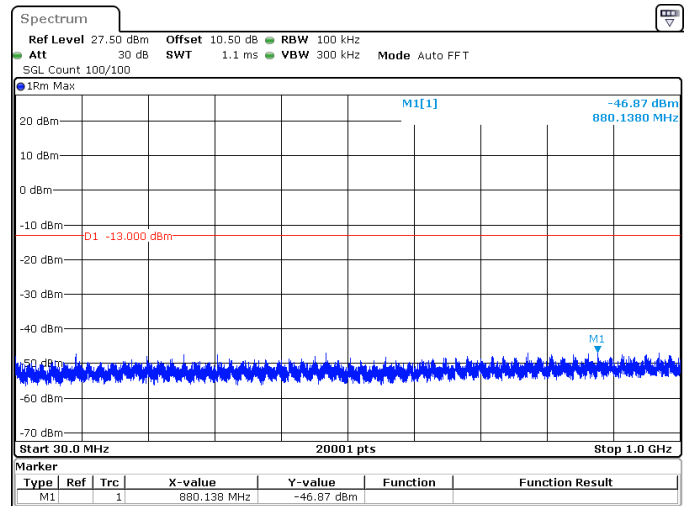
20MHz_15kHz_1770MHz_DFT-s-OFDM QPSK_RB100@0 -46.87 dBm
