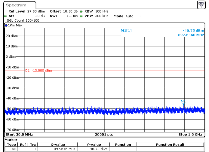
20MHz_15kHz_1745MHz_DFT-s-OFDM QPSK_RB1@0 -46.75 dBm
