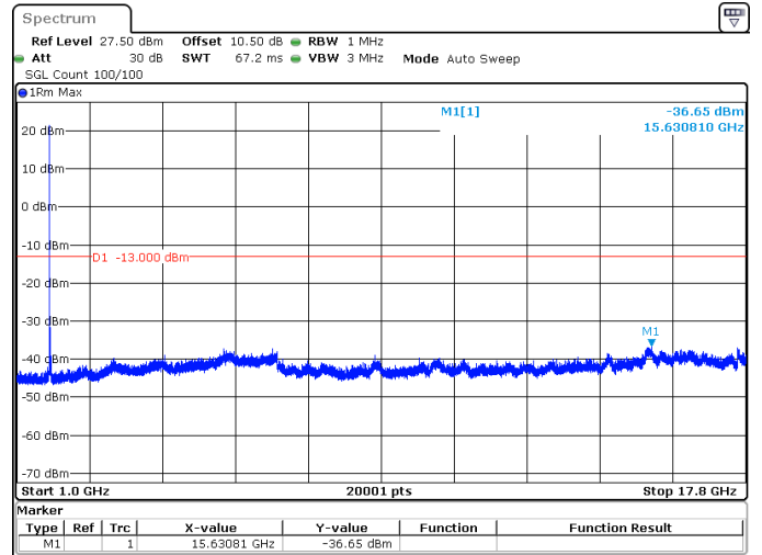
30MHz_15kHz_1765MHz_DFT-s-OFDM QPSK_RB1@0 -36.65 dBm
