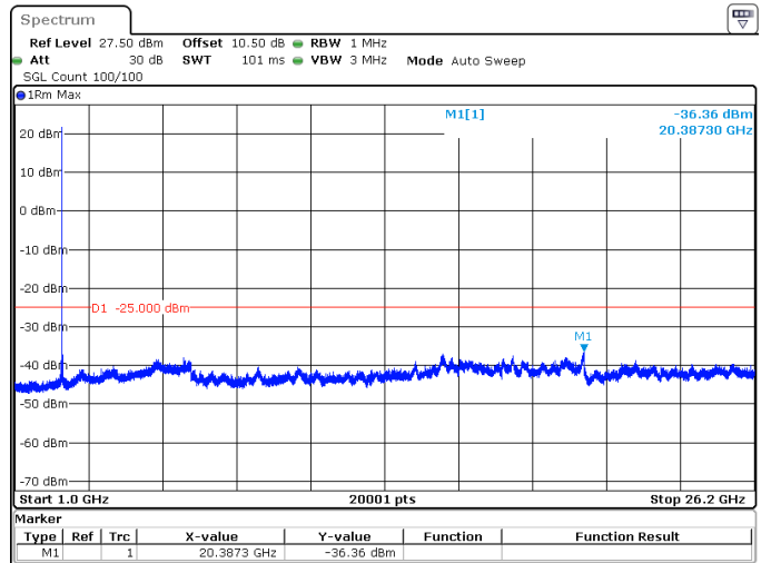
30MHz_30kHz_2585MHz_DFT-s-OFDM QPSK_RB1@77 -36.36 dBm
