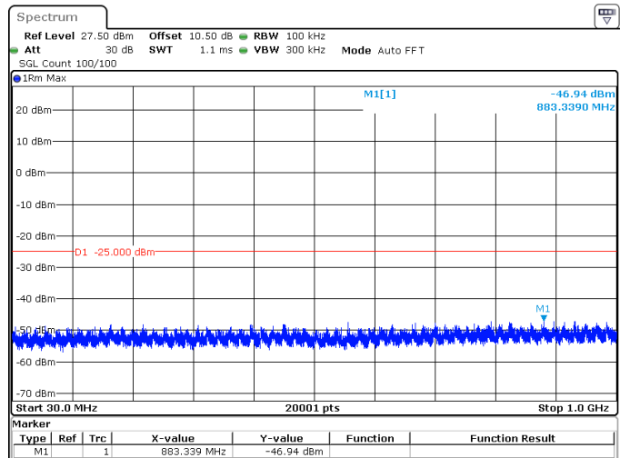
30MHz_30kHz_2585MHz_DFT-s-OFDM QPSK_RB75@0 -46.94 dBm
