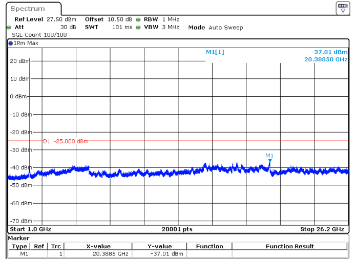
25MHz_30kHz_2595MHz_DFT-s-OFDM QPSK_RB1@0 -37.01 dBm
