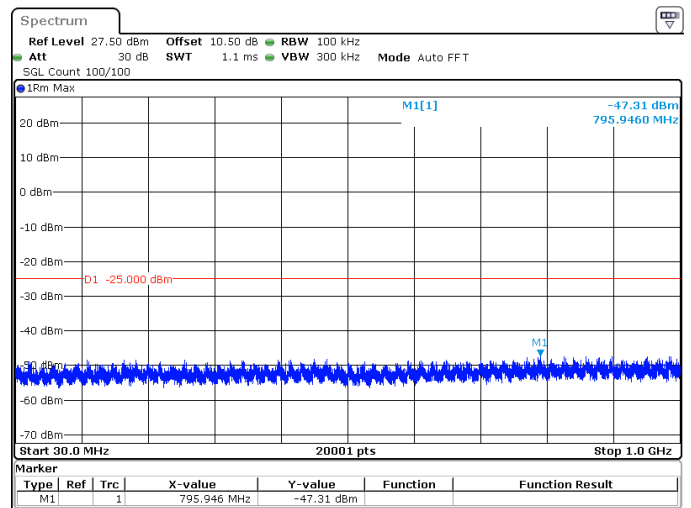
25MHz_30kHz_2582.5MHz_DFT-s-OFDM QPSK_RB64@0 -47.31 dBm
