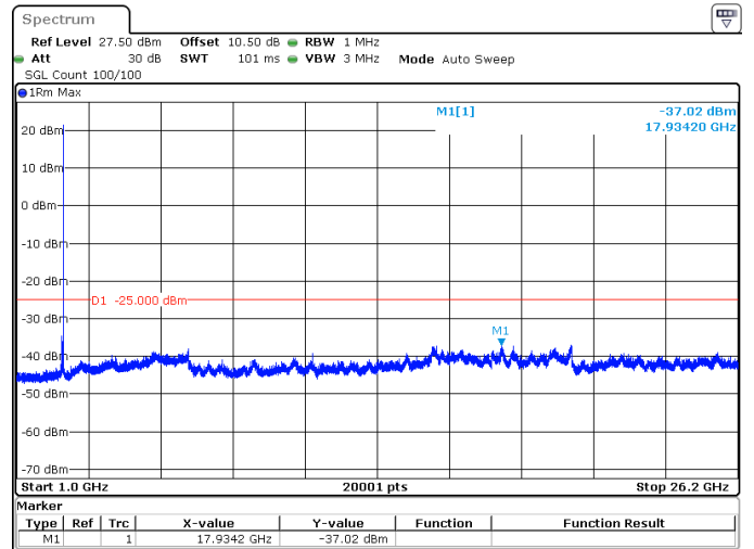
40MHz_30kHz_2595MHz_DFT-s-OFDM QPSK_RB1@105 -37.02 dBm
