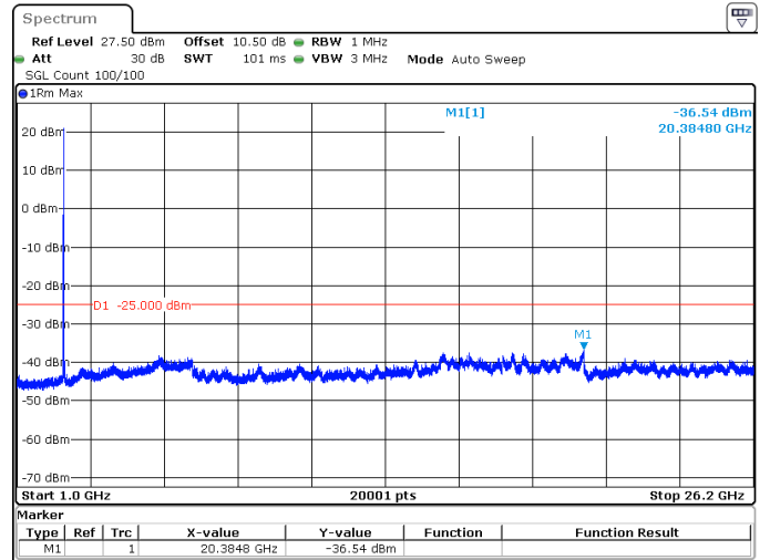
30MHz_30kHz_2595MHz_DFT-s-OFDM QPSK_RB1@0 -36.54 dBm
