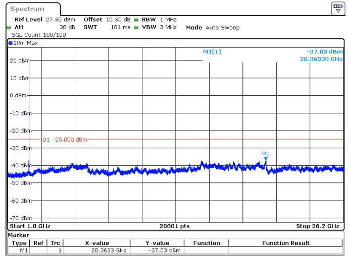
25MHz_30kHz_2582.5MHz_DFT-s-OFDM QPSK_RB1@64 -37.03 dBm
