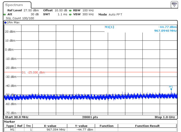
25MHz_30kHz_2607.5MHz_DFT-s-OFDM QPSK_RB64@0 -44.77 dBm
