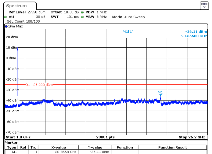
40MHz_30kHz_2595MHz_DFT-s-OFDM QPSK_RB100@0 -36.11 dBm
