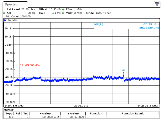
25MHz_30kHz_2595MHz_DFT-s-OFDM QPSK_RB64@0 -35.33 dBm
