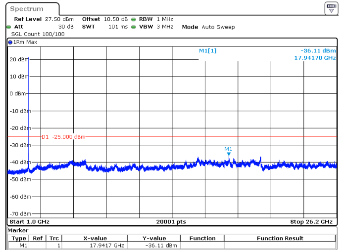
30MHz_30kHz_2595MHz_DFT-s-OFDM QPSK_RB1@77 -36.11 dBm
