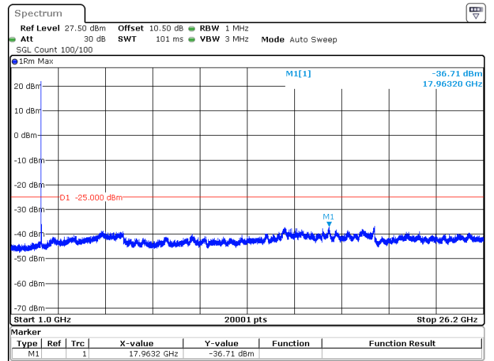
25MHz_30kHz_2607.5MHz_DFT-s-OFDM QPSK_RB1@0 -36.71 dBm
