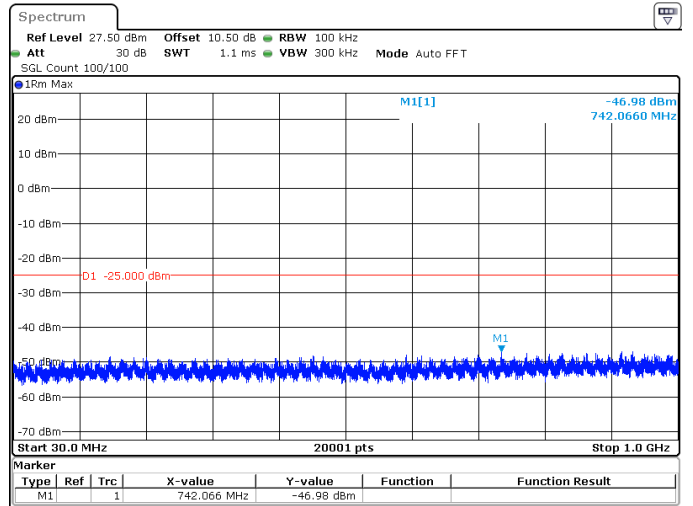
30MHz_30kHz_2585MHz_DFT-s-OFDM QPSK_RB1@0 -46.98 dBm
