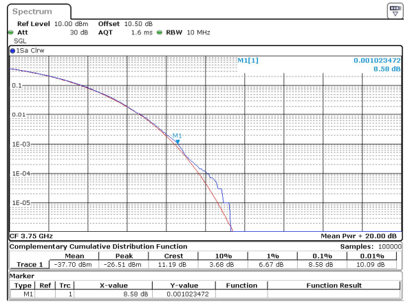
10MHz_30kHz_3750MHz_DFT-s-OFDM 16 QAM_RB24@0 8.58 dB
