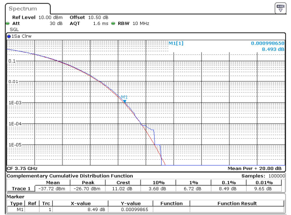
10MHz_30kHz_3750MHz_DFT-s-OFDM 64 QAM_RB24@0 8.49 dB
