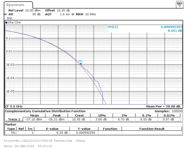
10MHz_30kHz_3500MHz_CP-OFDM QPSK_RB24@0 8.55 dB
