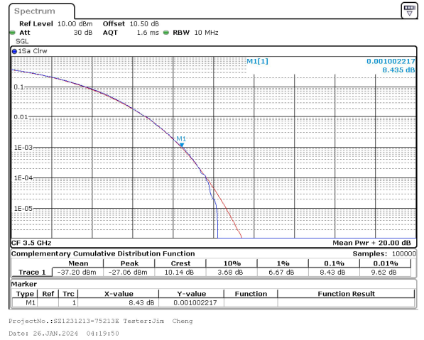
10MHz_15kHz_3500MHz_CP-OFDM QPSK_RB52@0 8.43 dB
