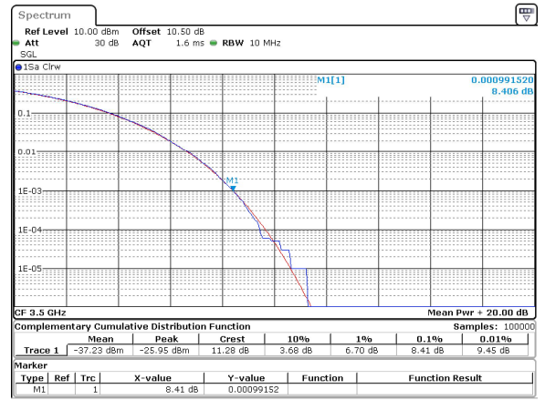
10MHz_15kHz_3500MHz_DFT-s-OFDM PI/2 BPSK_RB50@0 8.41 dB
