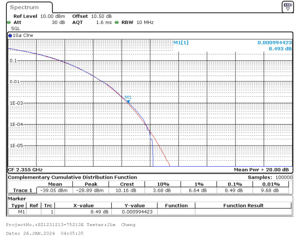
10MHz_30kHz_2355MHz_CP-OFDM 256 QAM_RB24@0 8.49 dB
