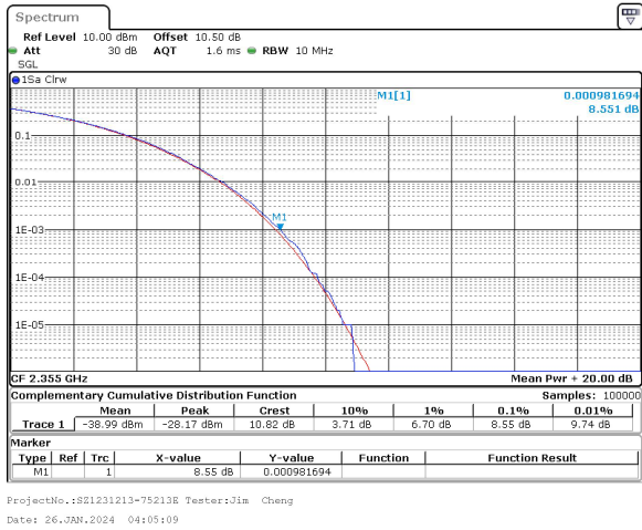
10MHz_30kHz_2355MHz_CP-OFDM 64 QAM_RB24@0 8.55 dB
