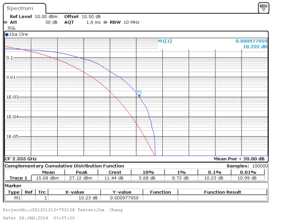
10MHz_30kHz_2355MHz_DFT-s-OFDM 16 QAM_RB24@0 10.23 dB
