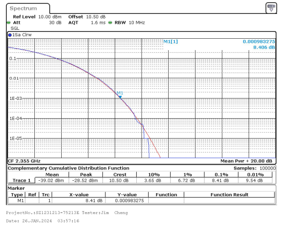
10MHz_30kHz_2355MHz_DFT-s-OFDM 256 QAM_RB24@0 8.41 dB
