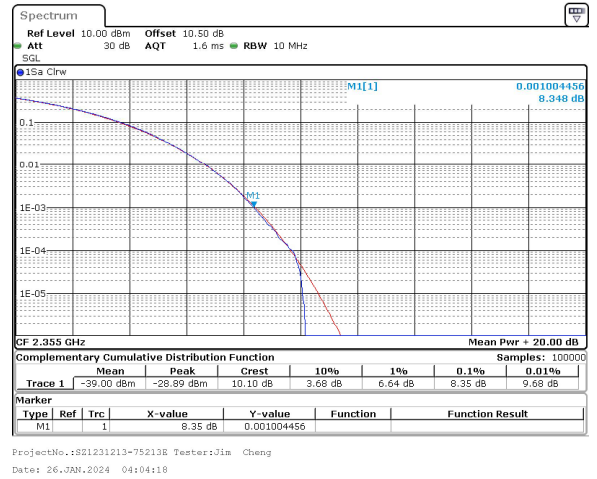
10MHz_30kHz_2355MHz_CP-OFDM QPSK_RB24@0 8.35 dB
