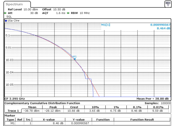
10MHz_30kHz_2595MHz_CP-OFDM 256 QAM_RB24@0 8.46 dB
