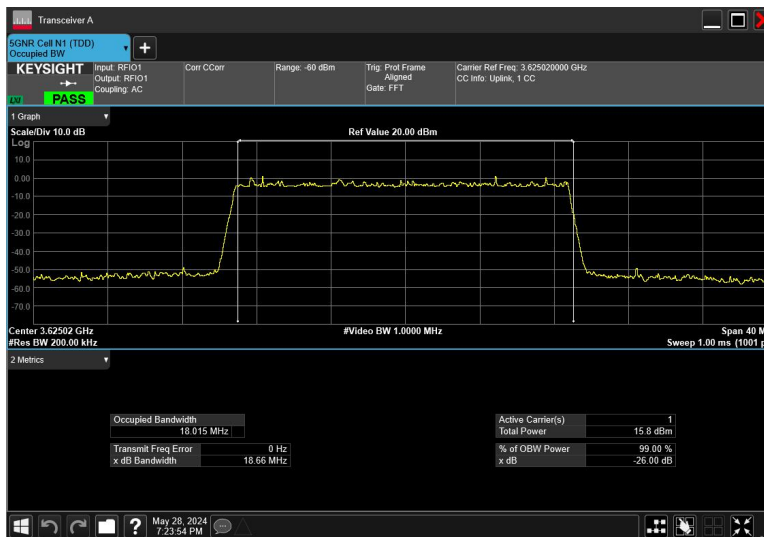
20MHz_30kHz_3625MHz_DFT-s-OFDM 256QAM_RB50@0
