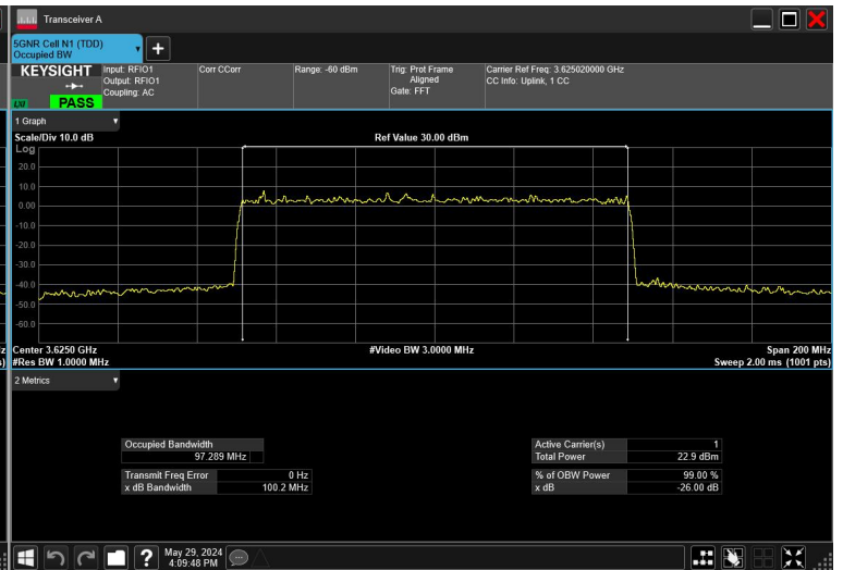
100MHz_30kHz_3625MHz_CP-OFDM QPSK_RB273@0
