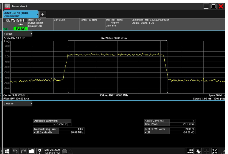
30MHz_30kHz_3625MHz_DFT-s-OFDM \pi/2 BPSK_RB75@0
