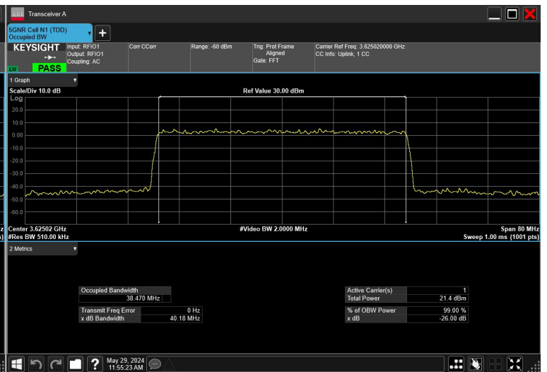
40MHz_15kHz_3625MHz_CP-OFDM QPSK_RB216@0
