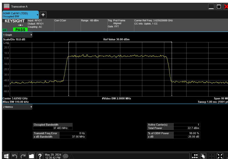
40MHz_30kHz_3625MHz_DFT-s-OFDM QPSK_RB100@0
