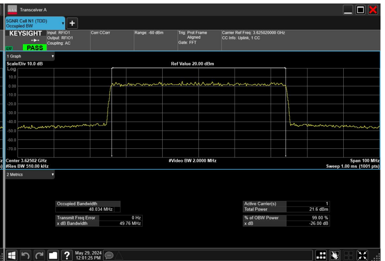
50MHz_15kHz_3625MHz_CP-OFDM QPSK_RB270@0
