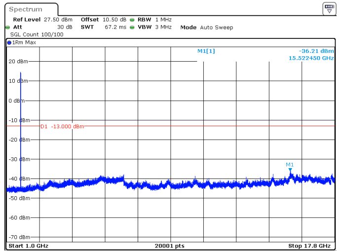
5MHz_15kHz_1712.5MHz_DFT-s-OFDM QPSK_RB25@0 -36.21 dBm
