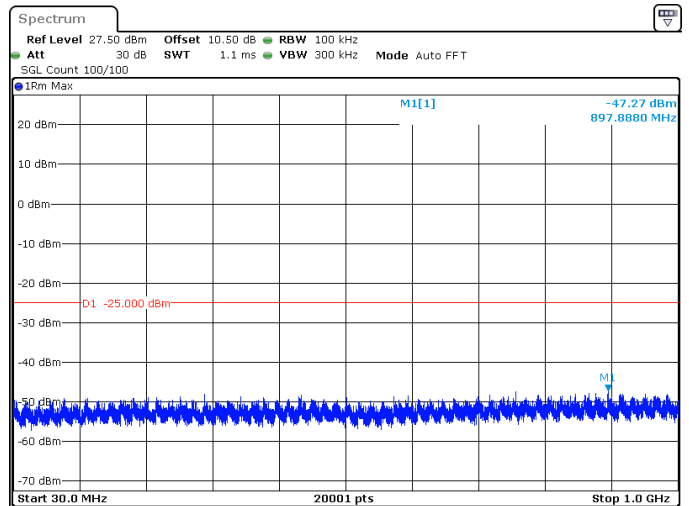
5MHz_15kHz_2502.5MHz_DFT-s-OFDM QPSK_RB25@0 -47.27 dBm
