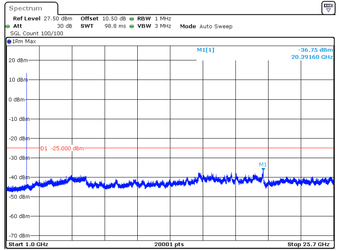
5MHz_15kHz_2502.5MHz_DFT-s-OFDM QPSK_RB1@0 -36.75 dBm
