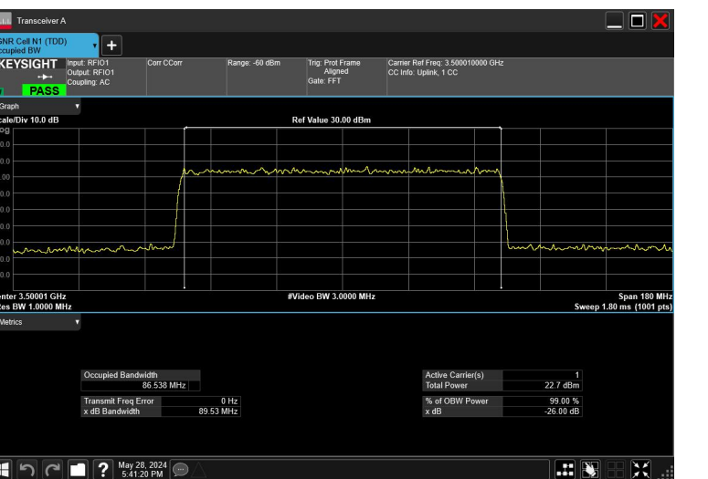
90MHz_30kHz_3500MHz_DFT-s-OFDM \pi/2 BPSK_RB243@0
