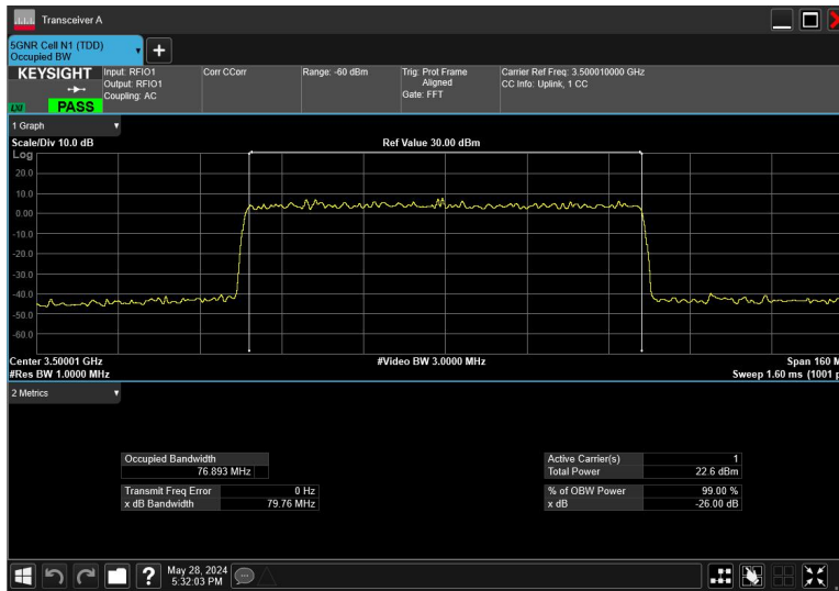
80MHz_30kHz_3500MHz_DFT-s-OFDM \pi/2 BPSK_RB216@0
