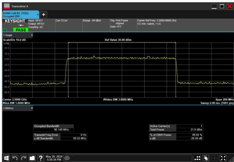
100MHz_30kHz_3500MHz_DFT-s-OFDM \pi/2 BPSK_RB270@0
