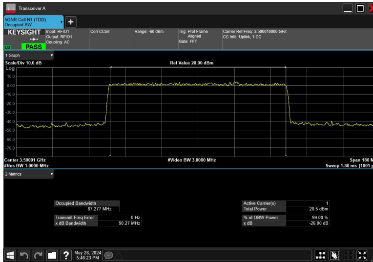
90MHz_30kHz_3500MHz_CP-OFDM QPSK_RB245@0
