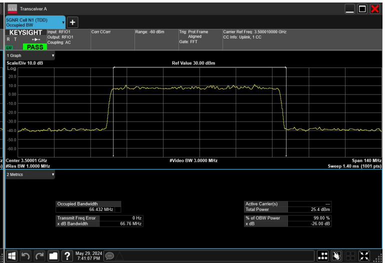
70MHz_30kHz_3500MHz_DFT-s-OFDM QPSK_RB180@0
