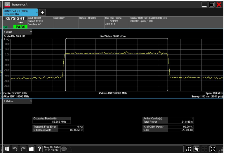
90MHz_30kHz_3500MHz_DFT-s-OFDM QPSK_RB243@0
