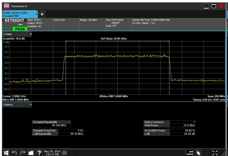
100MHz_30kHz_3500MHz_DFT-s-OFDM QPSK_RB270@0
