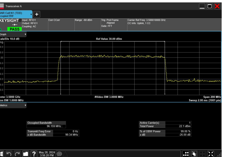
100MHz_30kHz_3500MHz_DFT-s-OFDM π/2 BPSK_RB270@0
