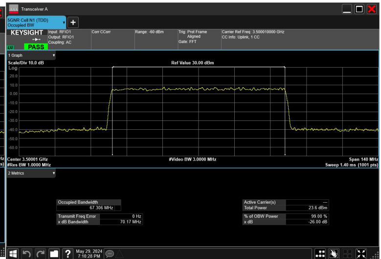
70MHz_30kHz_3500MHz_CP-OFDM QPSK_RB189@0
