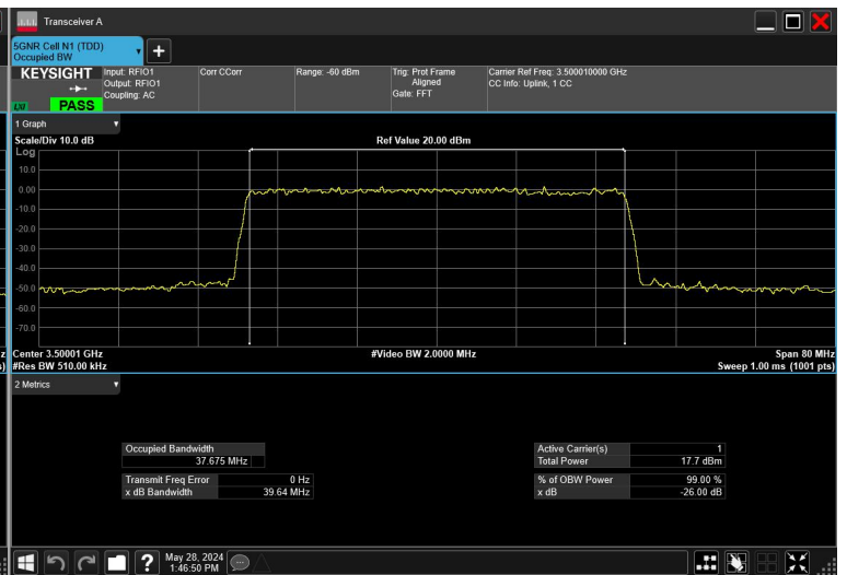
40MHz_30kHz_3500MHz_CP-OFDM QPSK_RB106@0
