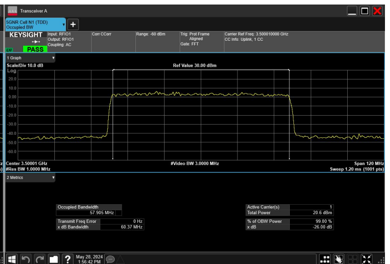
60MHz_30kHz_3500MHz_DFT-s-OFDM \pi/2 BPSK_RB162@0
