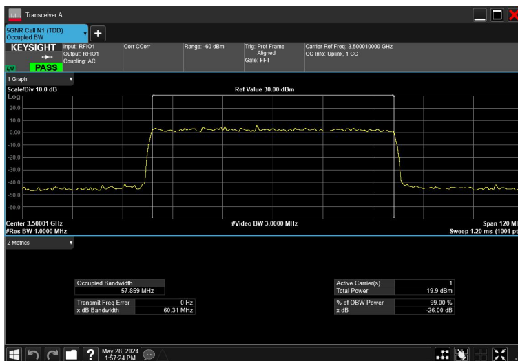
60MHz_30kHz_3500MHz_DFT-s-OFDM QPSK_RB162@0
