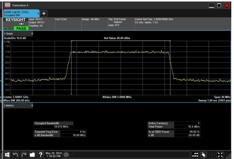
20MHz_30kHz_3500MHz_DFT-s-OFDM 16QAM_RB50@0
