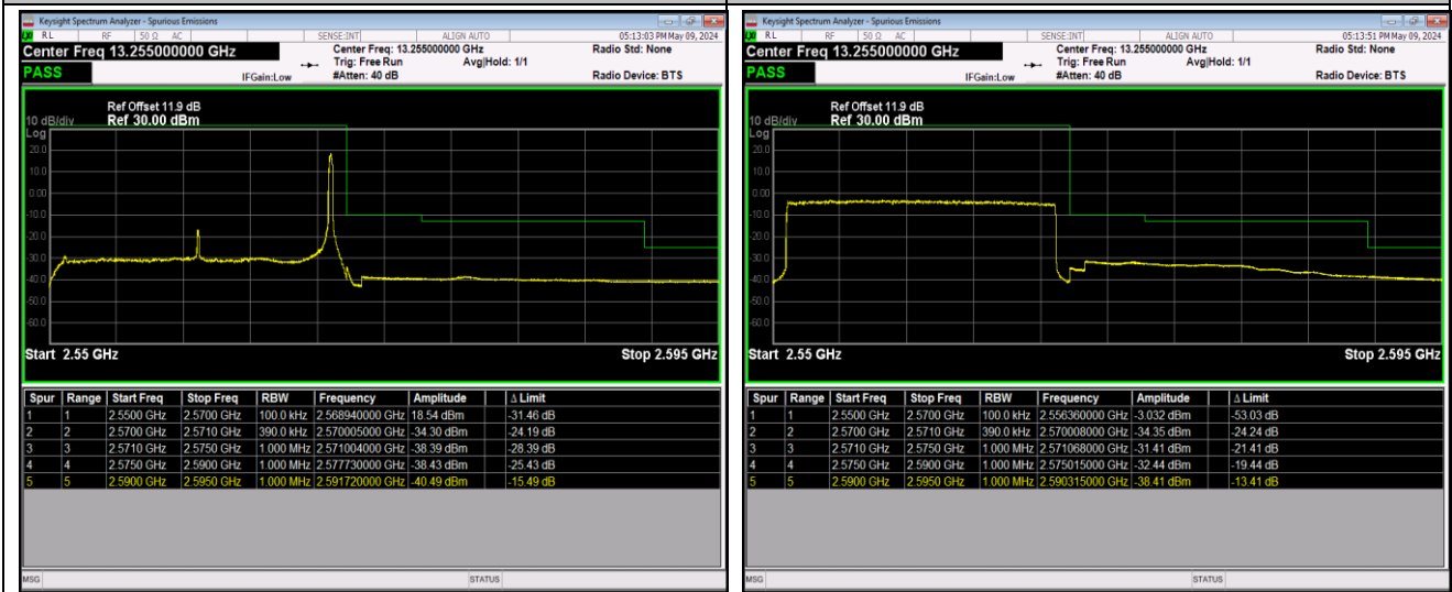
Band7_20MHz_16QAM_21350_1RB#99
