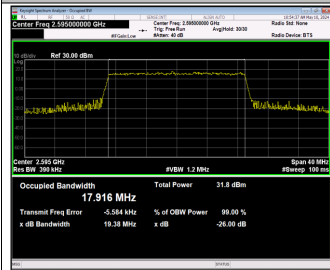
41(2535-2655)-20MHz-QPSK-40640-100RB#0-PASS
