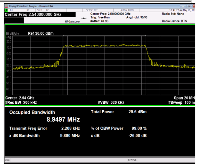
41(2535-2655)-10MHz-64QAM-40090-50RB#0-PASS
