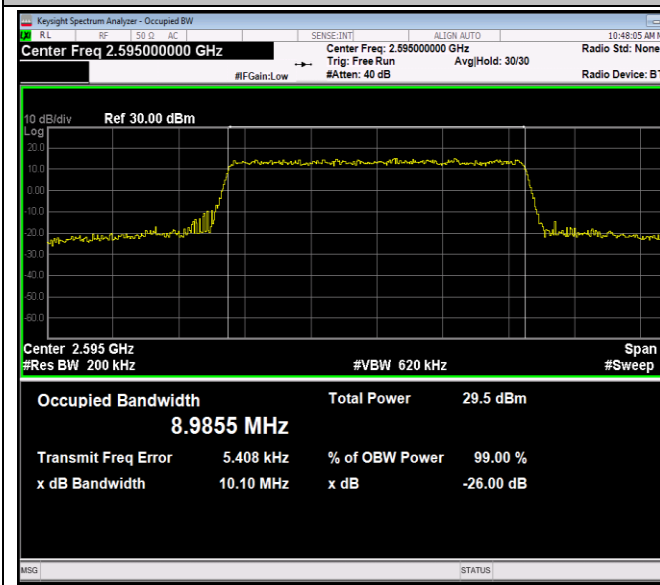
41(2535-2655)-10MHz-64QAM-40640-50RB#0-PASS
