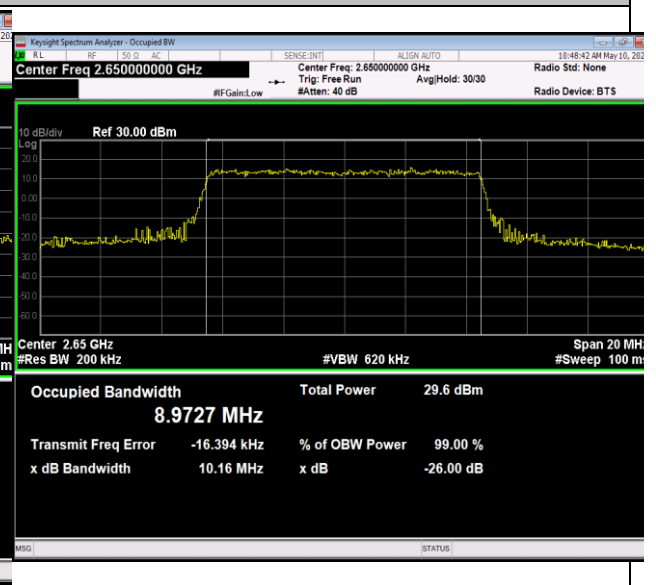
41(2535-2655)-10MHz-64QAM-41190-50RB#0-PASS
