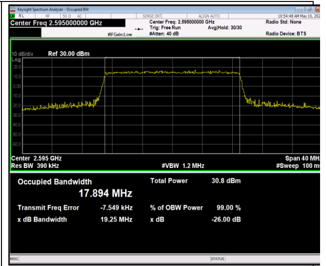
41(2535-2655)-20MHz-16QAM-40640-100RB#0-PASS
