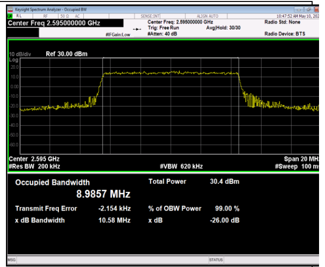
41(2535-2655)-10MHz-16QAM-40640-50RB#0-PASS
