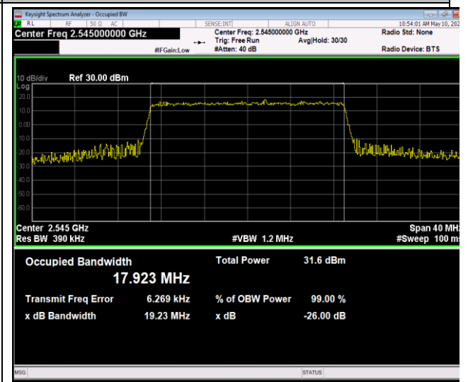
41(2535-2655)-20MHz-QPSK-40140-100RB#0-PASS
