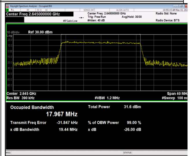
41(2535-2655)-20MHz-QPSK-41140-100RB#0-PASS
