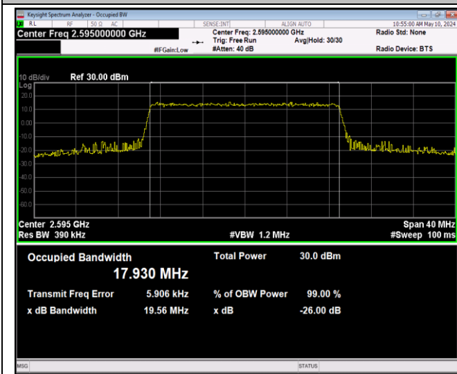
41(2535-2655)-20MHz-64QAM-40640-100RB#0-PASS
