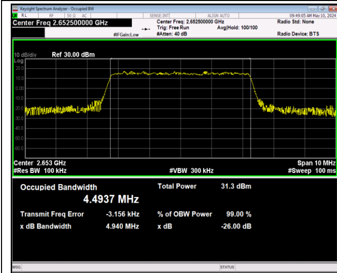
41(2535-2655)-5MHz-QPSK-41215-25RB#0-PASS
