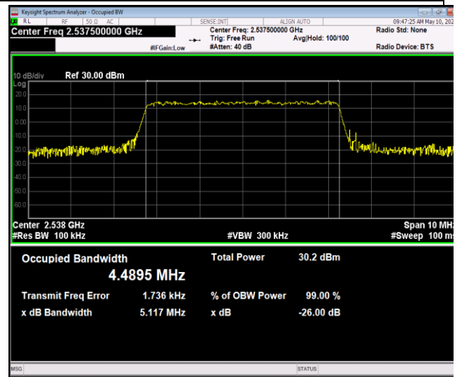
41(2535-2655)-5MHz-16QAM-40065-25RB#0-PASS
