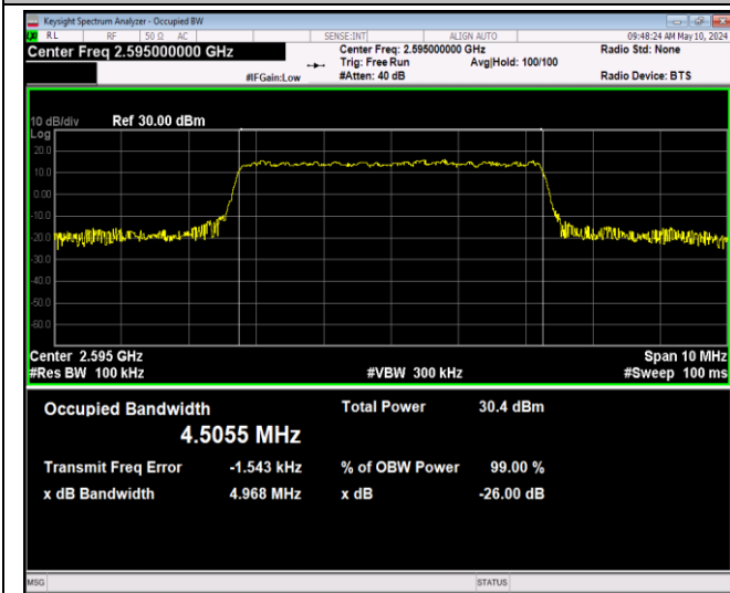
41(2535-2655)-5MHz-16QAM-40640-25RB#0-PASS
