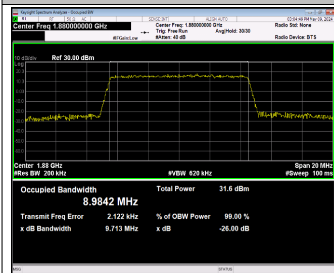
Band2-10MHz-QPSK-18900-50RB#0-PASS
