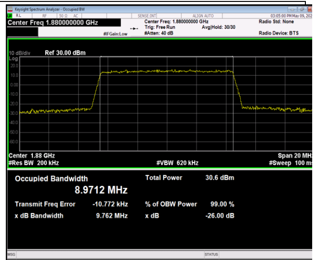
Band2-10MHz-16QAM-18900-50RB#0-PASS
