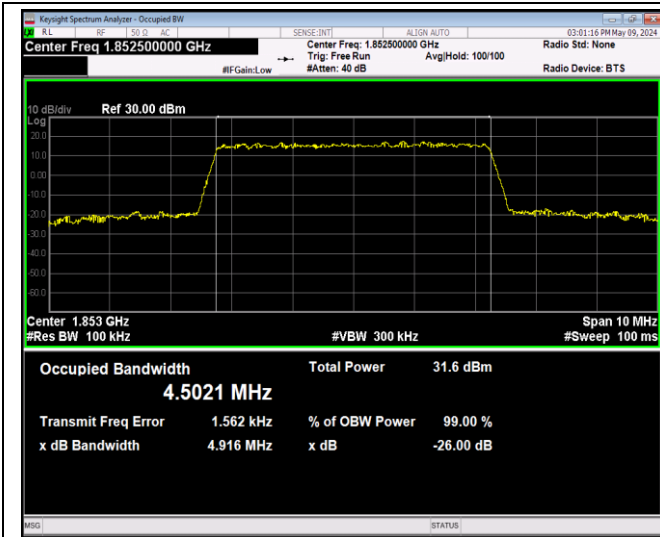
Band2-5MHz-QPSK-18625-25RB#0-PASS
