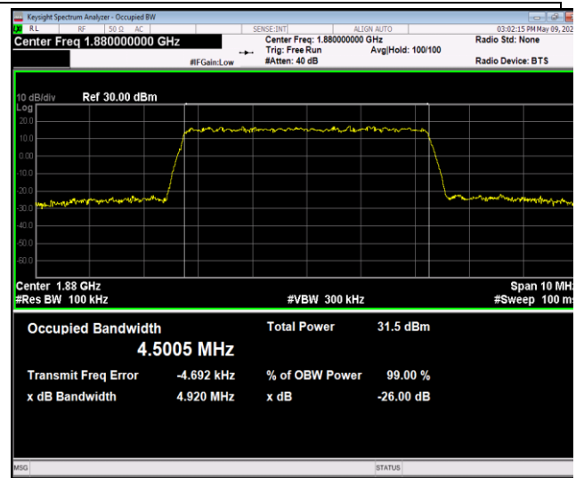
Band2-5MHz-QPSK-18900-25RB#0-PASS
