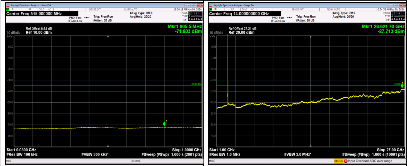
Band7_20MHz_QPSK_21350_1RB#0_1000~27000_1000~27000
