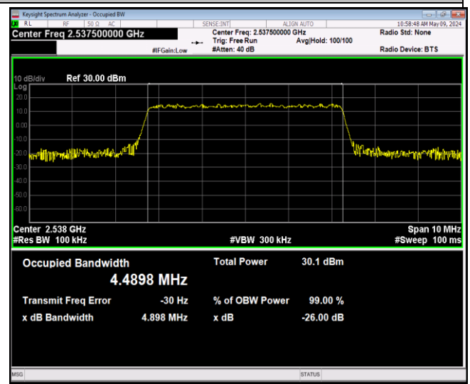
41(2535-2655)-5MHz-16QAM-40065-25RB#0-PASS
