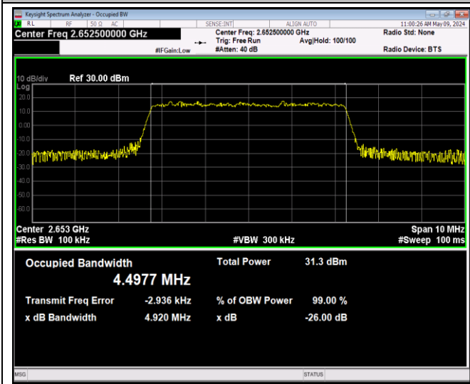
41(2535-2655)-5MHz-QPSK-41215-25RB#0-PASS
