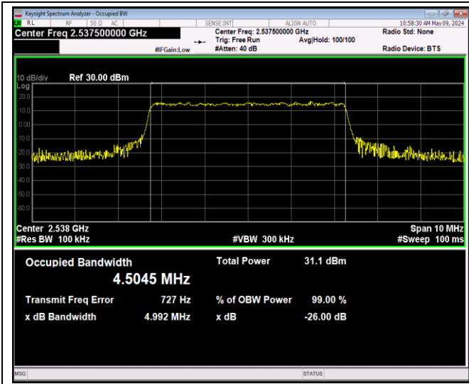
41(2535-2655)-5MHz-QPSK-40065-25RB#0-PASS
