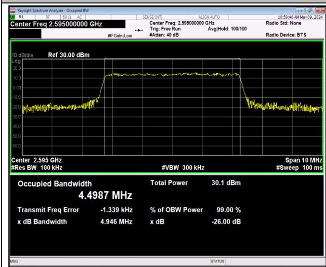
41(2535-2655)-5MHz-16QAM-40640-25RB#0-PASS
