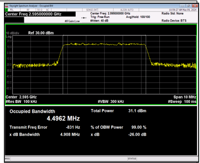
41(2535-2655)-5MHz-QPSK-40640-25RB#0-PASS
