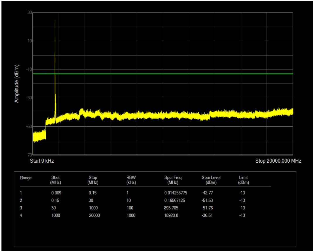
n66 SCS=15kHz DFT_QPSK BW=40MHz Channel=346000 RB=1 @215
