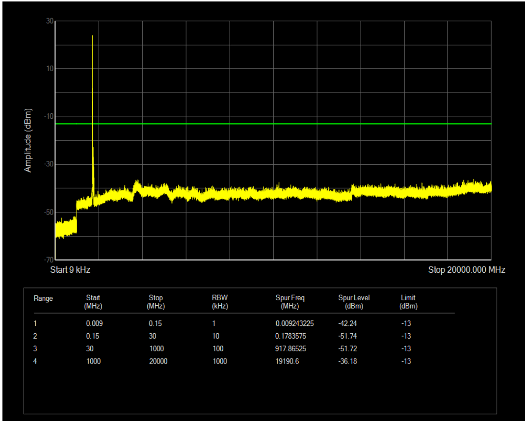
n66 SCS=15kHz DFT_QPSK BW=40MHz Channel=349000 RB=1 @215
