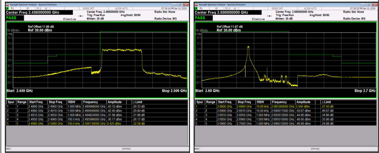
Band41-5MHz-16QAM-41565-1RB#24
