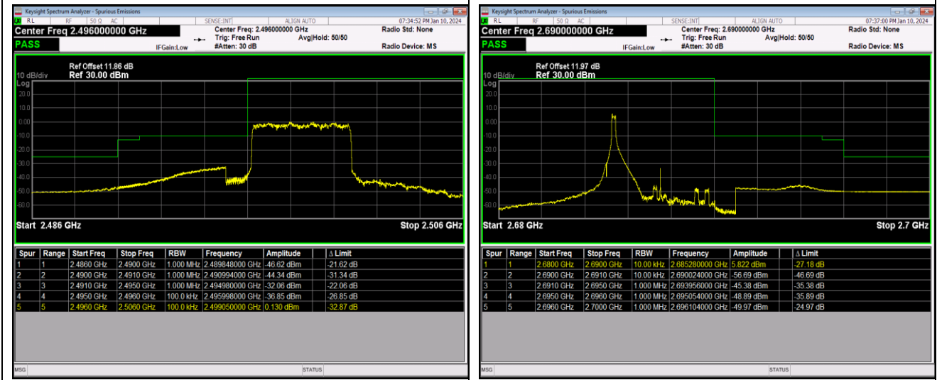
Band41-5MHz-64QAM-41565-1RB#24
