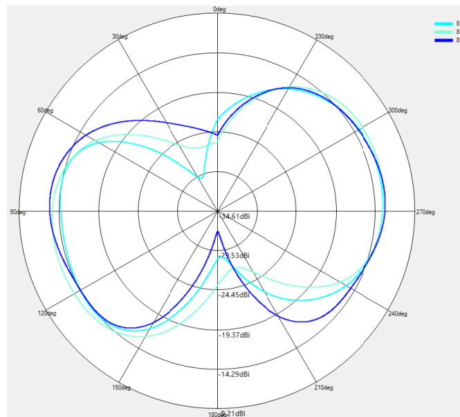
GSM850/ WCDMA B5/LTE B5/B20 Theta=0deg
