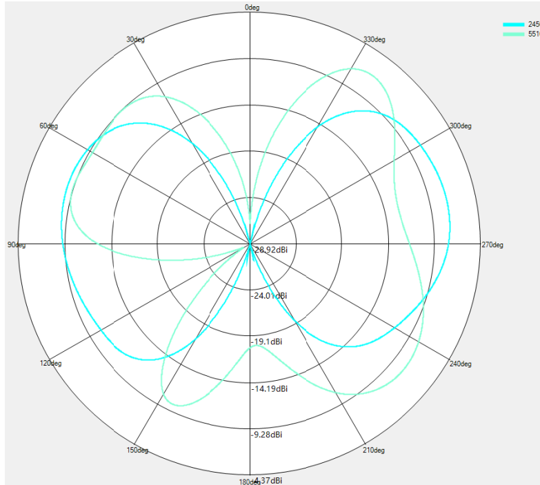
2.4G/5G WIFI&BT Phi=90deg
