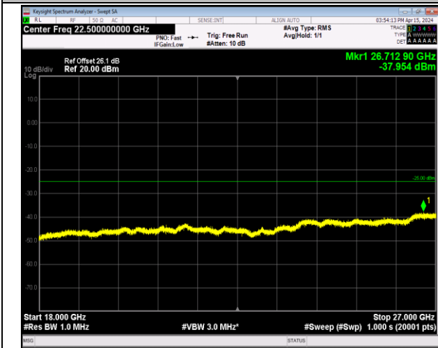
Band7_20MHz_16QAM_20850_1RB#0_18000~27000_18 000~27000
