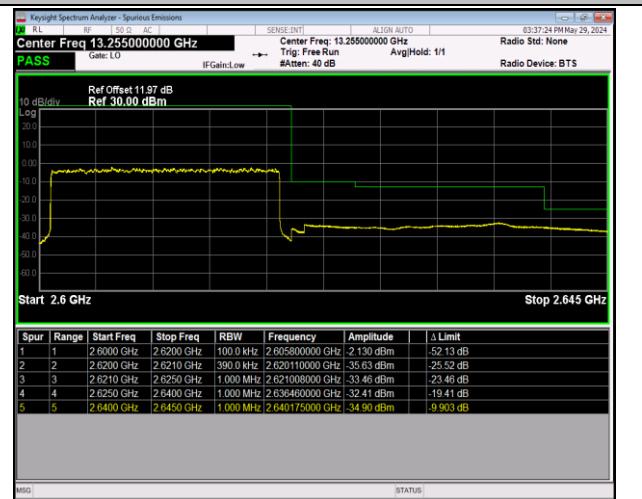
Band38_20MHz_QPSK_38150_1RB#99
