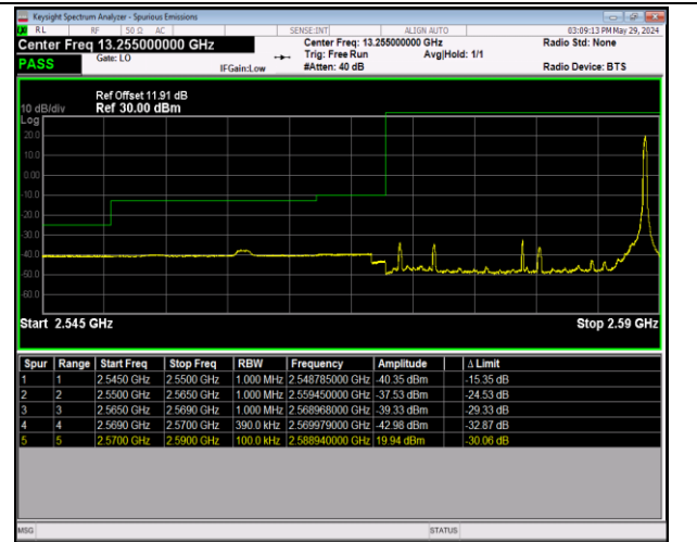
Band38_20MHz_QPSK_37850_1RB#99
