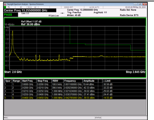
Band38_20MHz_QPSK_37850_100RB#99
