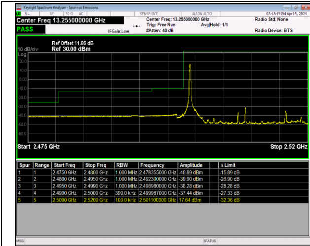
Band7_20MHz_16QAM_2085_1RB#0
