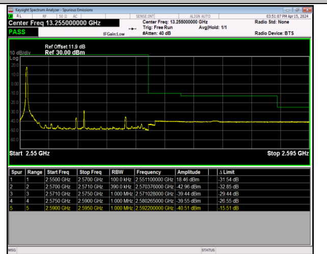
Band7_20MHz_16QAM_21350_1RB#0
