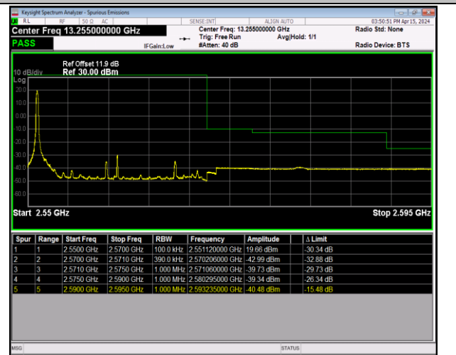
Band7_20MHz_QPSK_21350_1RB#0
