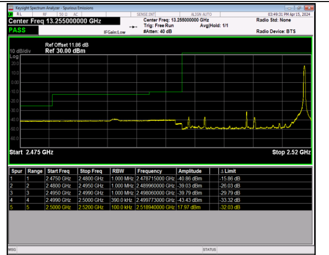
Band7_20MHz_16QAM_2085_1RB#99
