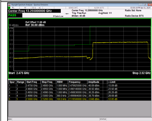
Band7_20MHz_16QAM_2085_100RB#0
