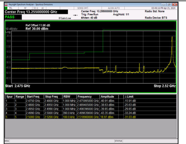
Band7_20MHz_QPSK_20850_1RB#99
