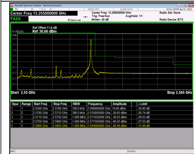
Band7_20MHz_QPSK_21350_1RB#99
