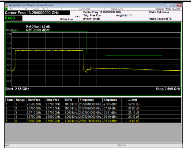
Band7_20MHz_QPSK_21350_100RB#0
