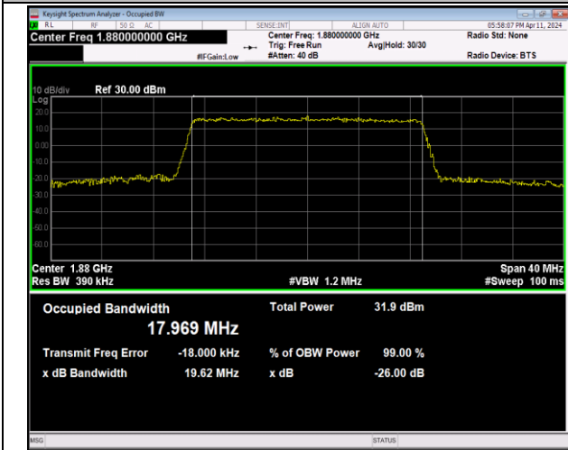
Band2-20MHz-QPSK-18900-100RB#0-PASS
