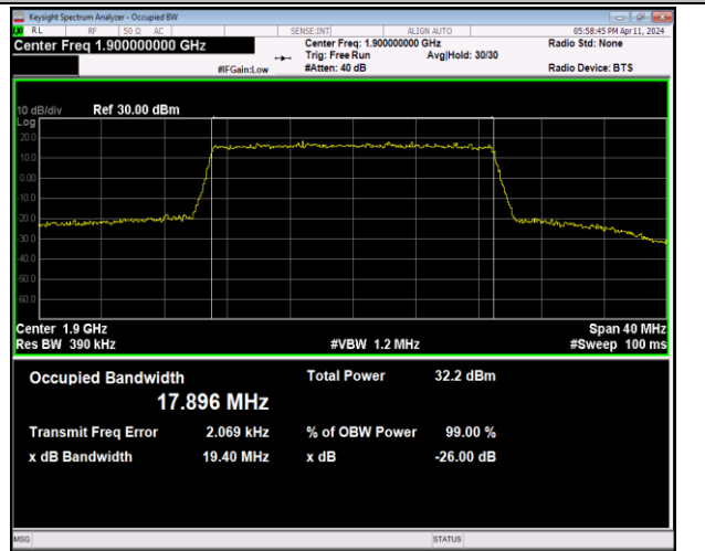
Band2-20MHz-QPSK-19100-100RB#0-PASS
