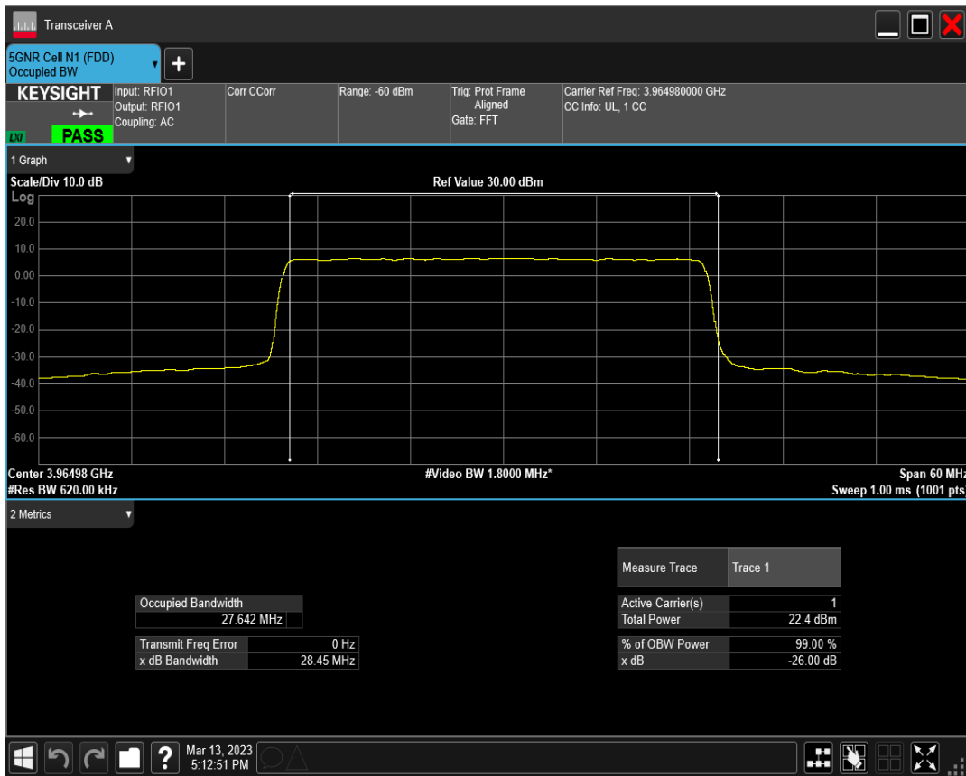
n77(3700-3980) SCS=30kHz CP_QPSK BW=30MHz Channel=664332 RB=78@0
