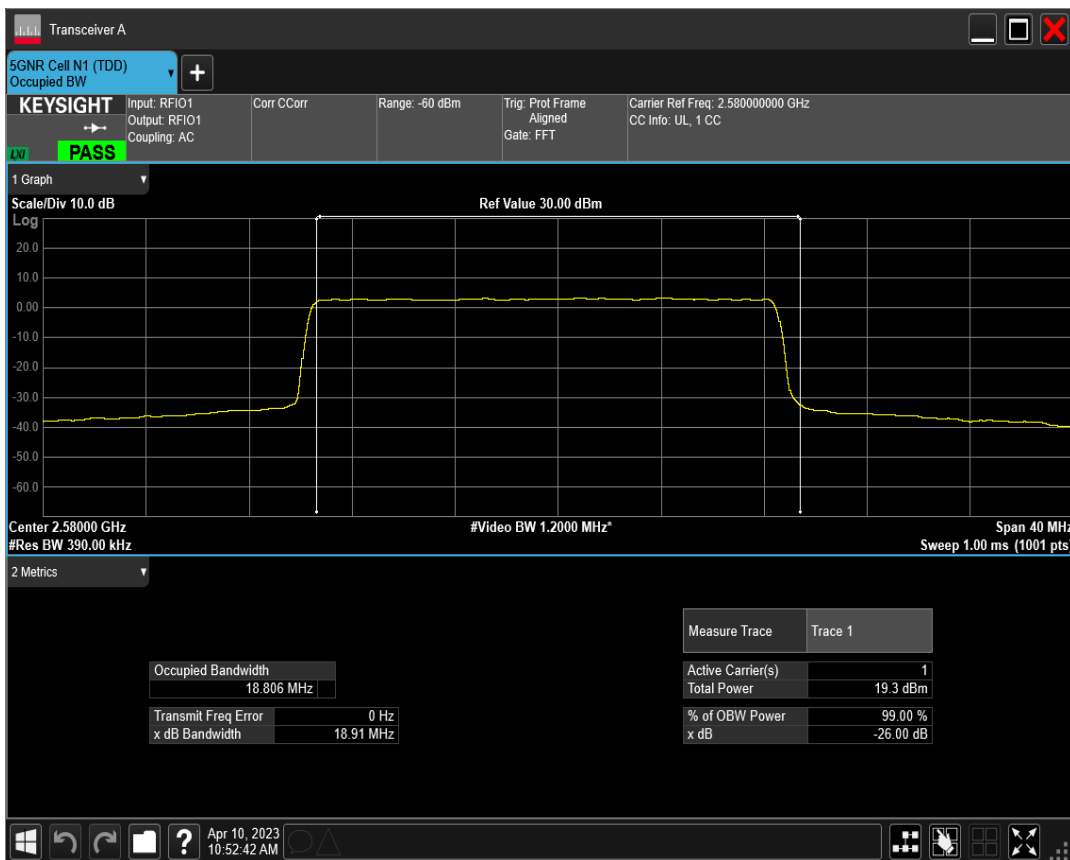
n38 SCS=15kHz CP_QPSK BW=20MHz Channel=516000 RB=106@0
