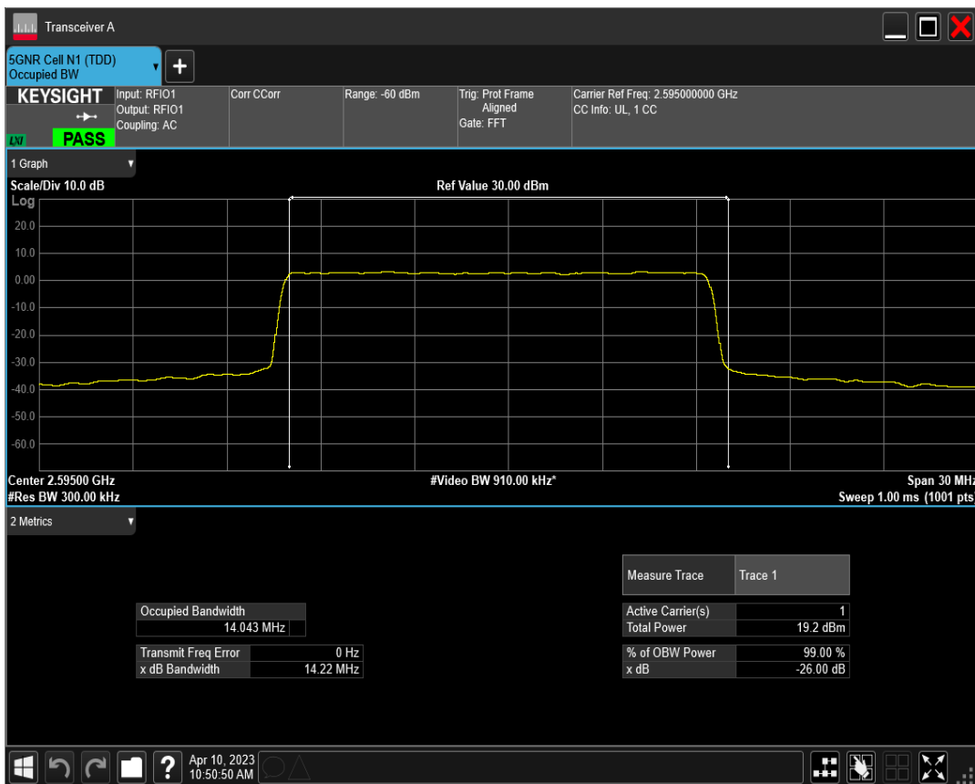
n38 SCS=15kHz CP_QPSK BW=15MHz Channel=519000 RB=79@0
