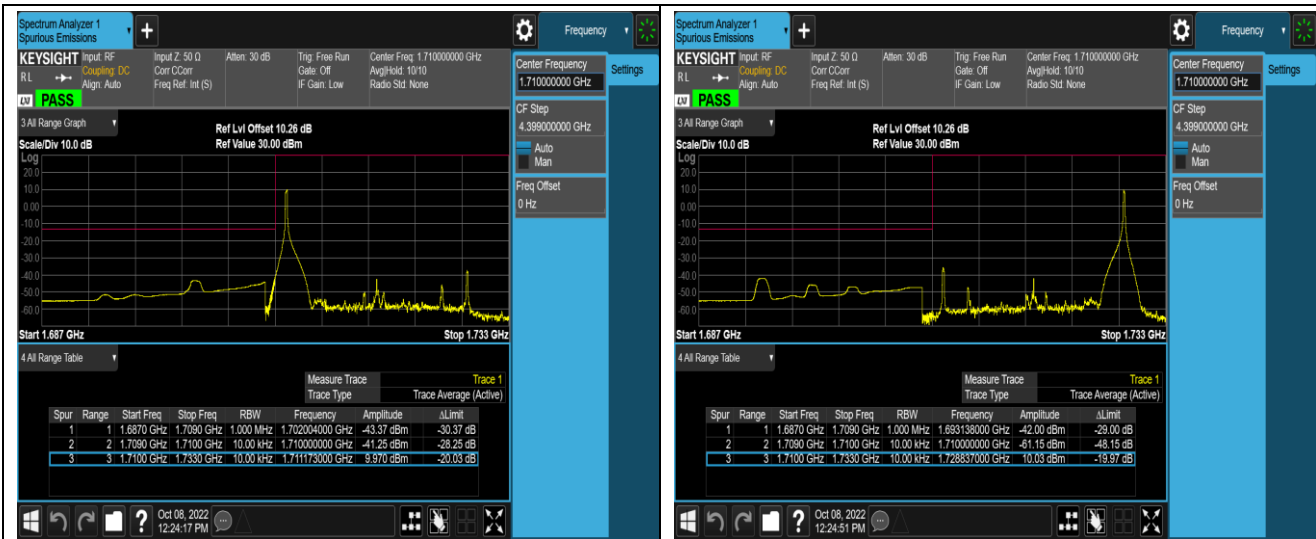
Band4-20MHz-QPSK-20050-100RB#0
