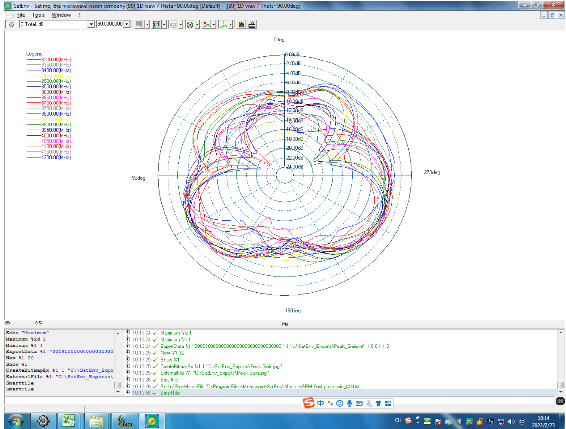
N77/N78 Theta=90deg
