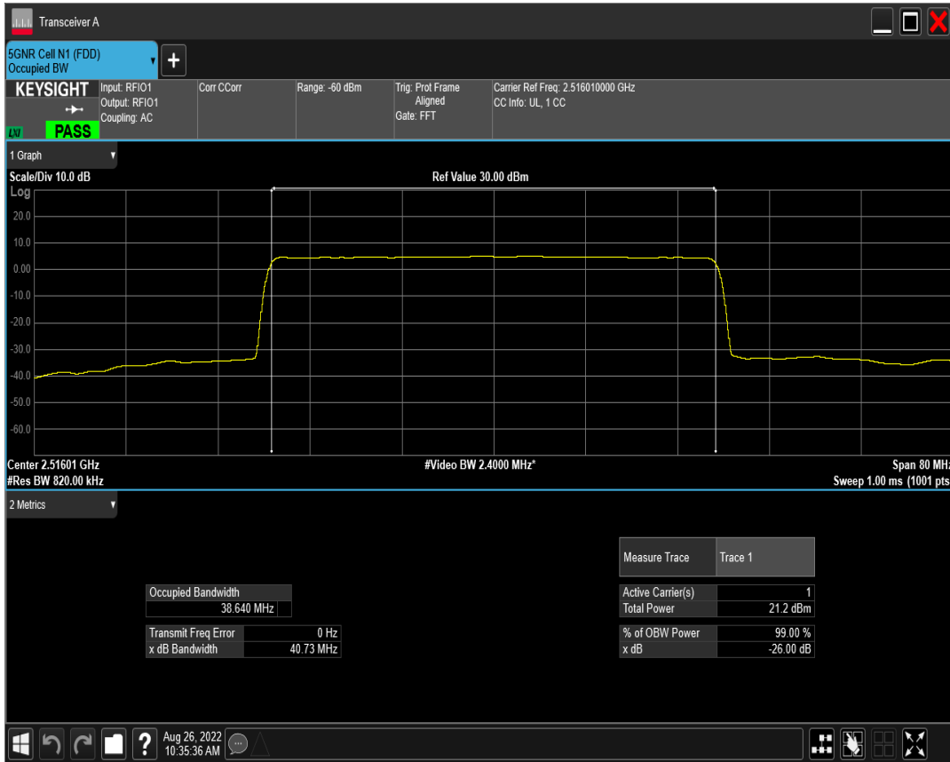
n41 SCS=15kHz CP_QPSK BW=40MHz Channel=503202 RB=216@0
