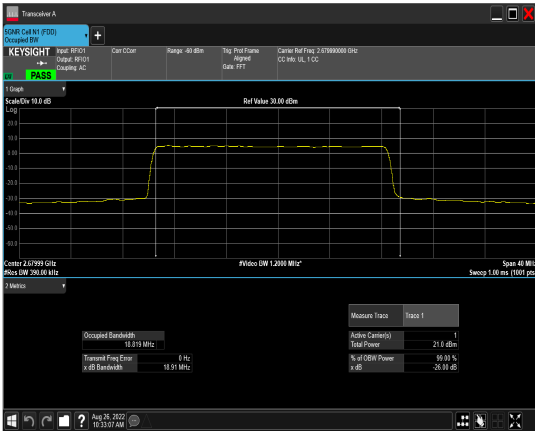
n41 SCS=15kHz CP_QPSK BW=20MHz Channel=535998 RB=106@0
