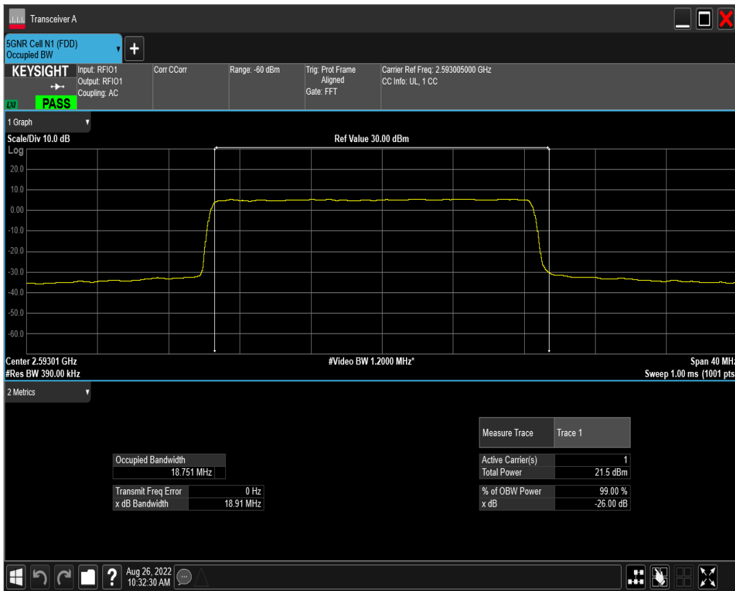
n41 SCS=15kHz CP_QPSK BW=20MHz Channel=518601 RB=106@0
