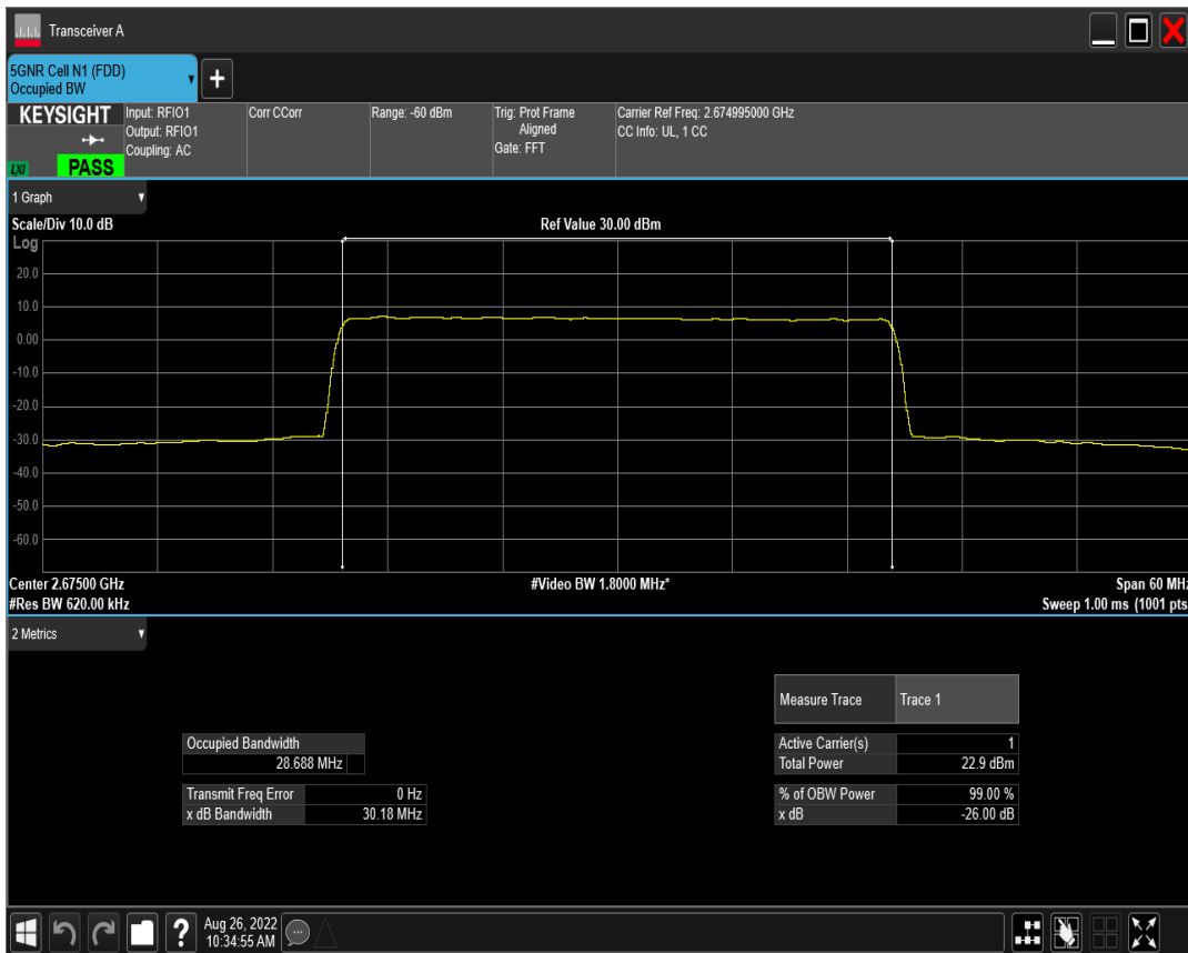
n41 SCS=15kHz DFT_QAM256 BW=30MHz Channel=534999 RB=160@0
