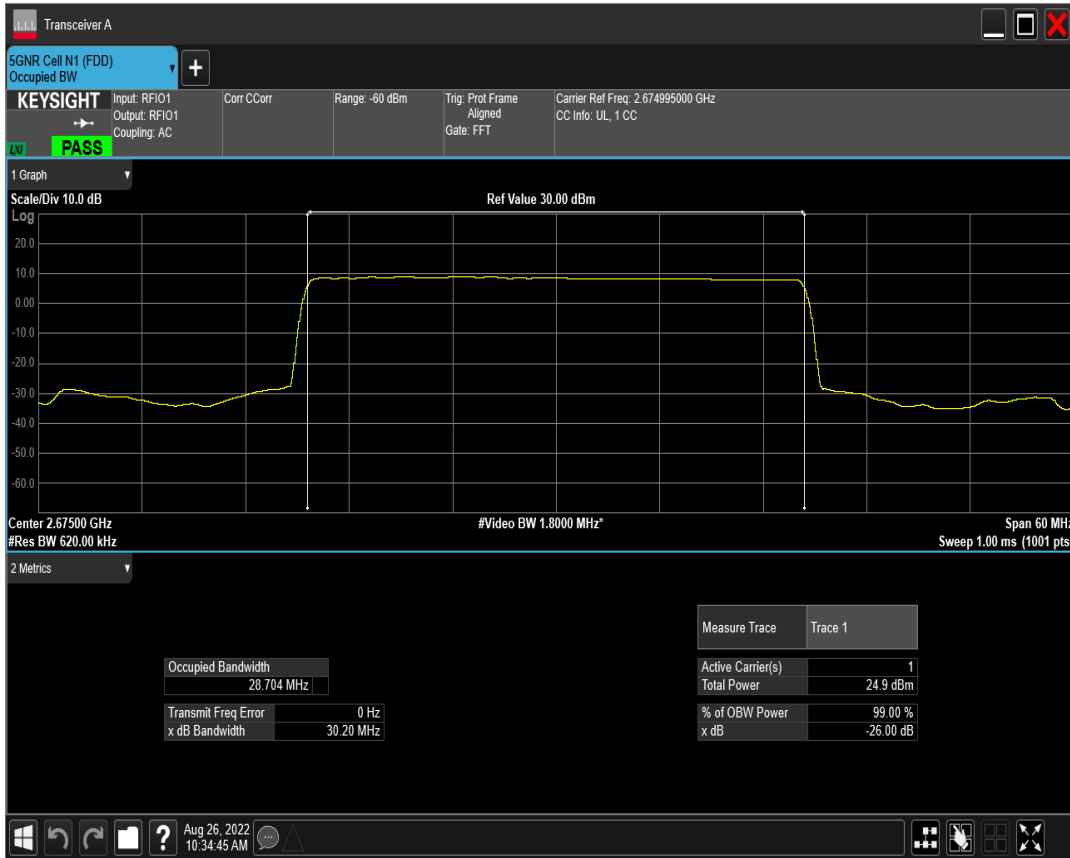
n41 SCS=15kHz DFT_QPSK BW=30MHz Channel=534999 RB=160@0
