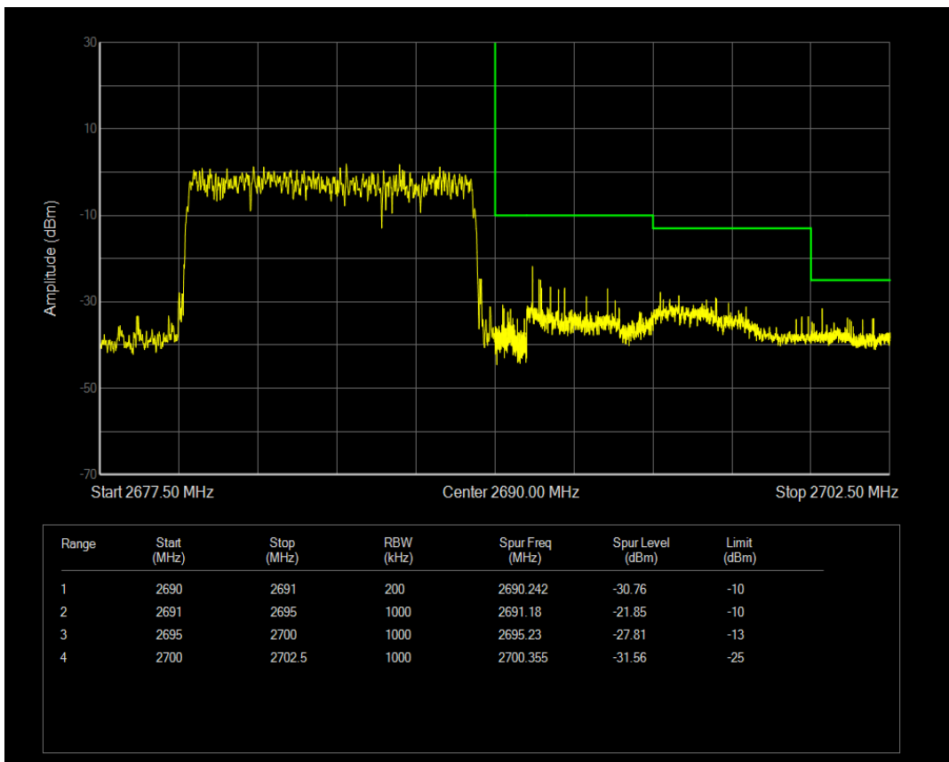
n41 SCS=15kHz DFT_QPSK BW=10MHz Channel=537000 RB=1@51
