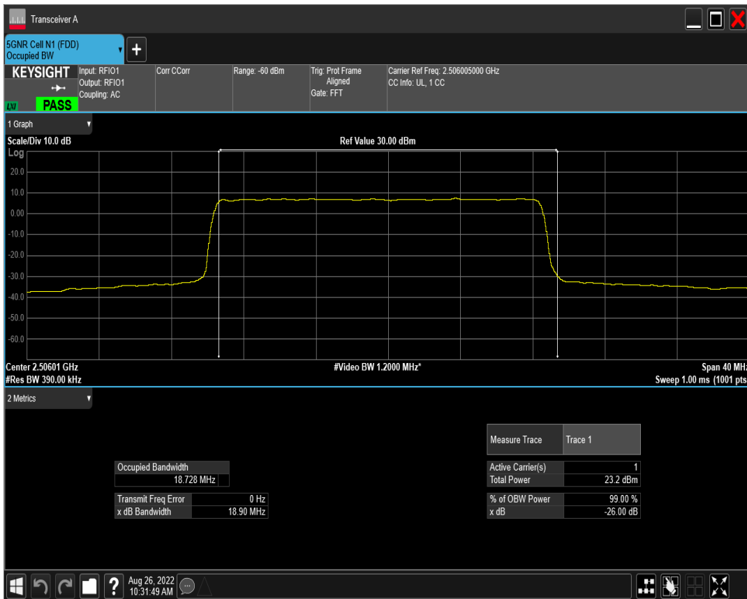
n41 SCS=15kHz DFT_QAM256 BW=20MHz Channel=501201 RB=100@0
