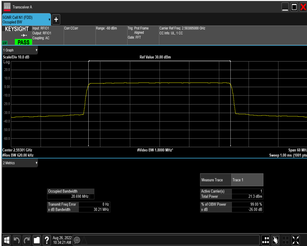
n41 SCS=15kHz CP_QPSK BW=30MHz Channel=518601 RB=160@0
