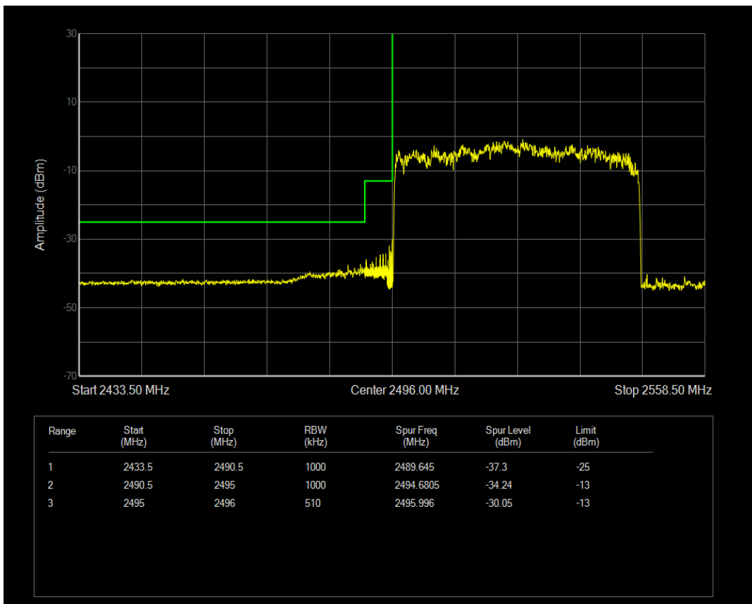
n41 SCS=15kHz DFT_QPSK BW=50MHz Channel=504201 RB=1@0
