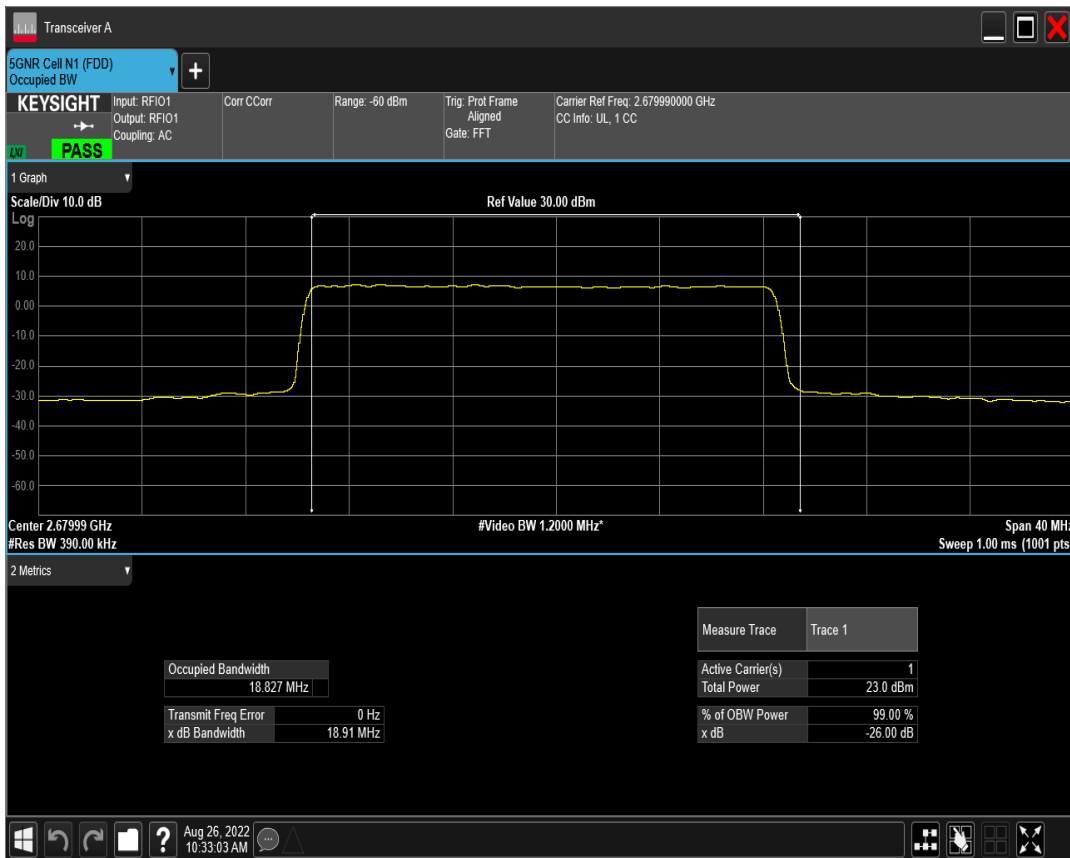
n41 SCS=15kHz DFT_QAM256 BW=20MHz Channel=535998 RB=100@0
